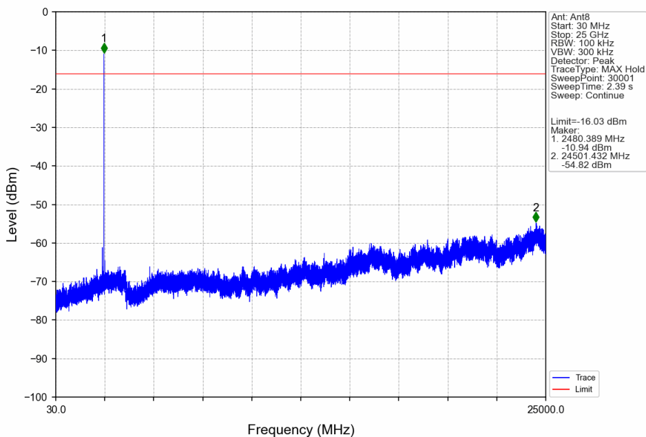
2M_HCH_2480MHz_Ant8_NTNV
