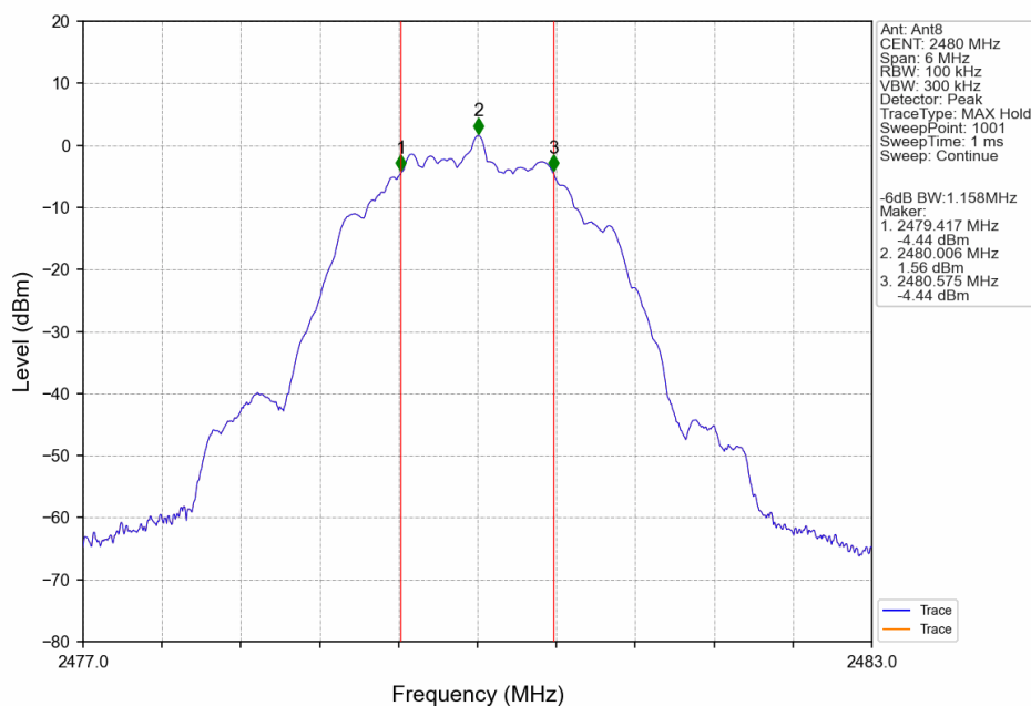
2M_HCH_2480MHz_Ant8_NTNV
