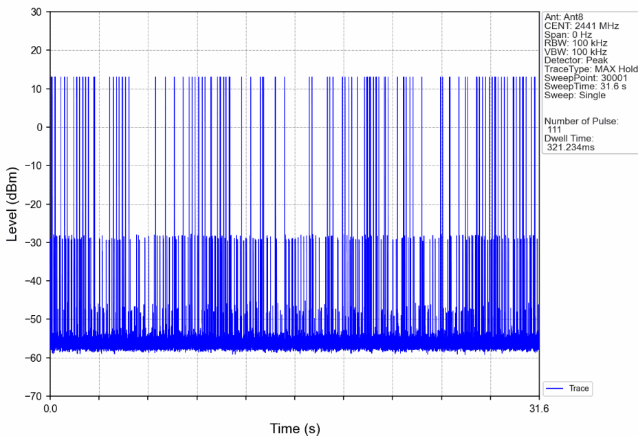
Pi/4DQPSK_2DH5_HOPP_Ant8_NTNV
