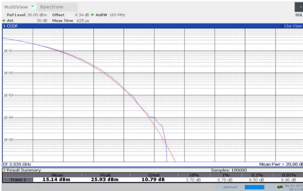
n7, CP-QPSK (PAPR)
