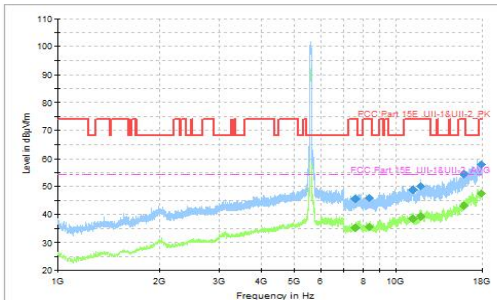
Fig. 70 Transmitter Spurious Emission (802.11be-EHT80, CH122 5610MHz, 1GHz-18GHz), MIMO
