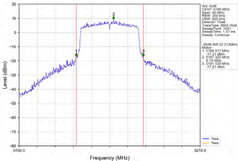
802.11ax(HEW20)_LCH_5180MHz_RU242_Left_Ant8_NTNV
