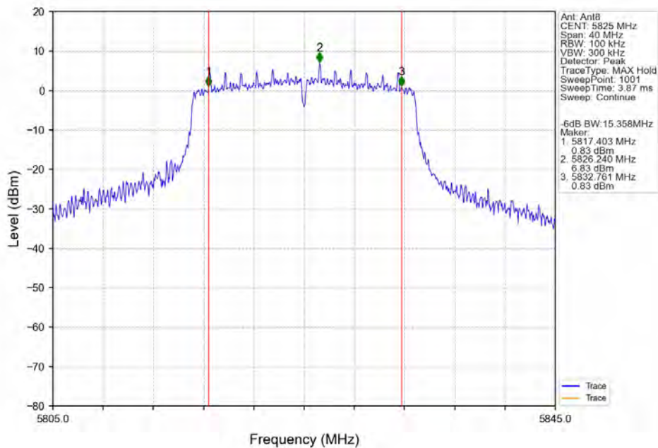
802.11n(HT20)_HCH_5825MHz_Ant8_NTNV
