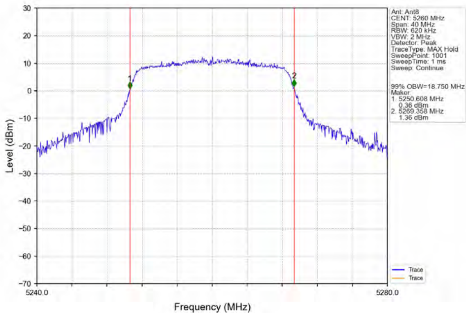
802.11n(HT20)_LCH_5260MHz_Ant8_NTNV
