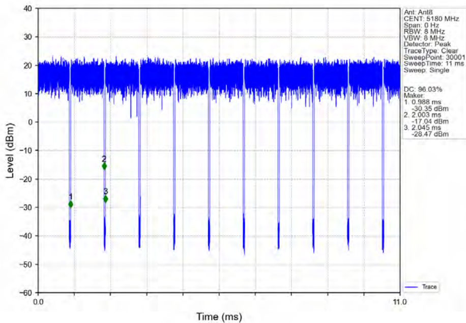
802.11ax(HEW20)_LCH_5180MHz_RU242_Left_Ant8_NTNV
