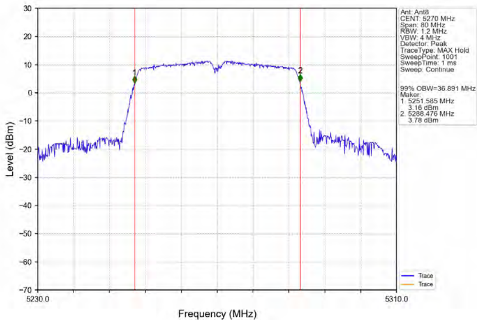
802.11ac(VHT40)_LCH_5270MHz_Ant8_NTNV
