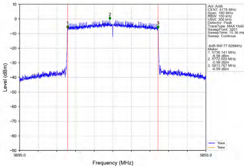
802.11ax(HEW80)_MCH_5775MHz_RU996_Left_Ant8_NTNV
