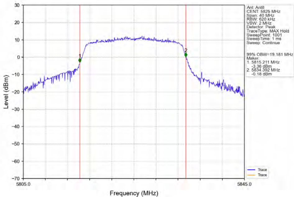
802.11n(HT20)_HCH_5825MHz_Ant8_NTNV
