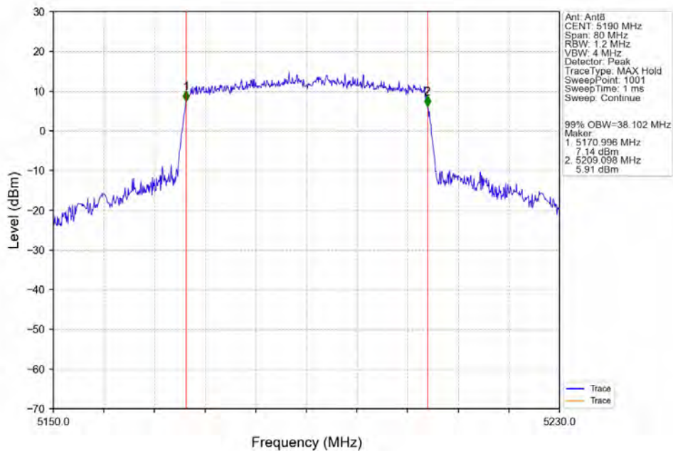
802.11ax(HEW40)_LCH_5190MHz_RU484_Left_Ant8_NTNV
