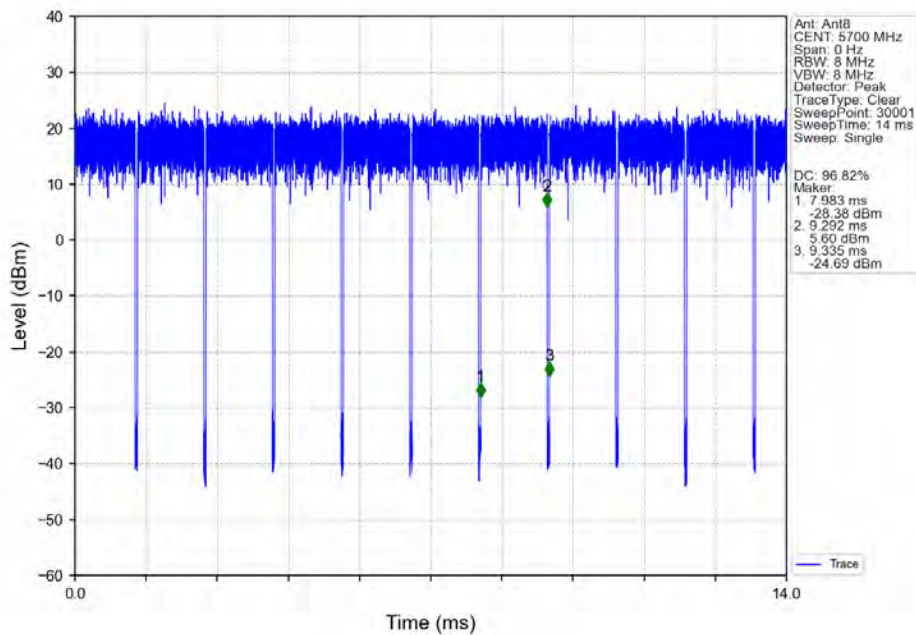
802.11ac(VHT20)_HCH_5700MHz_Ant8_NTNV
