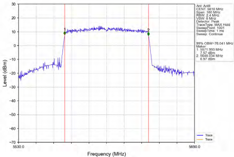
802.11ac(VHT80)_HCH_5610MHz_Ant8_NTNV
