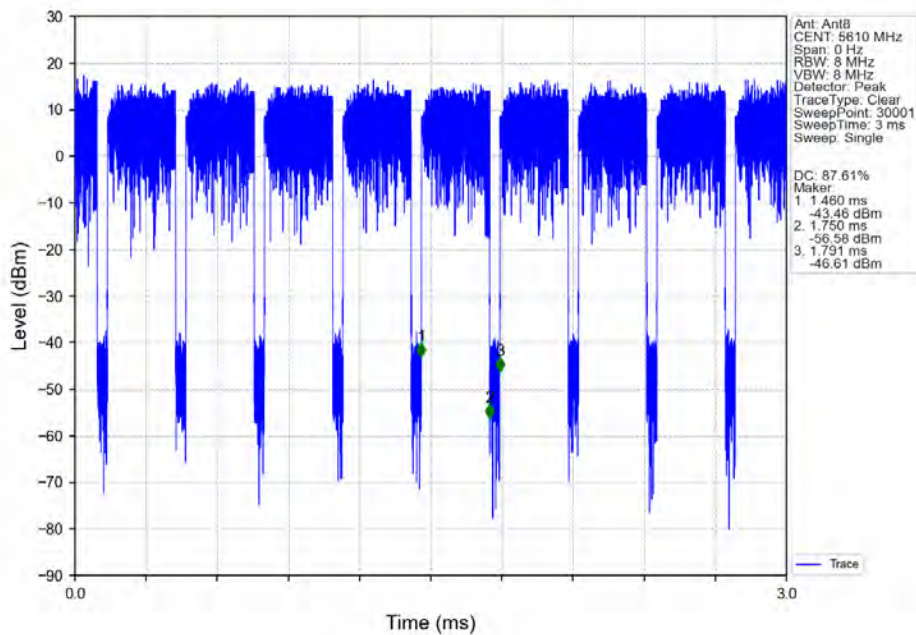
802.11ax(HEW80)_HCH_5610MHz_RU996_Left_Ant8_NTNV
