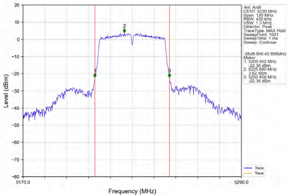
802.11n(HT40)_HCH_5230MHz_Ant8_NTNV
