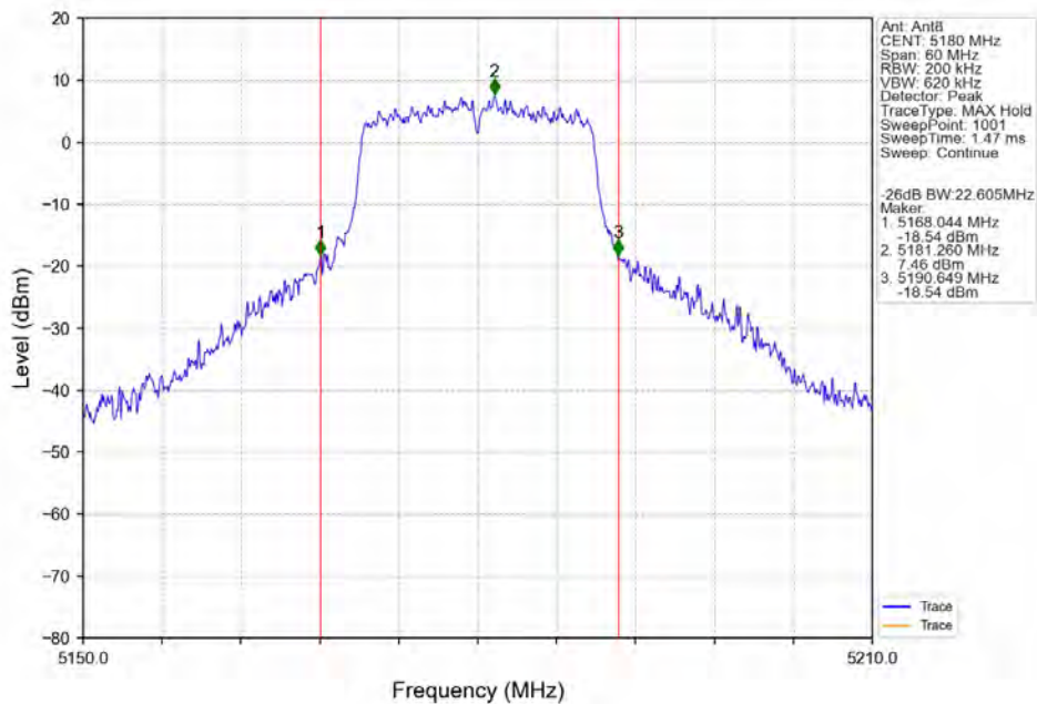
802.11n(HT20)_LCH_5180MHz_Ant8_NTNV
