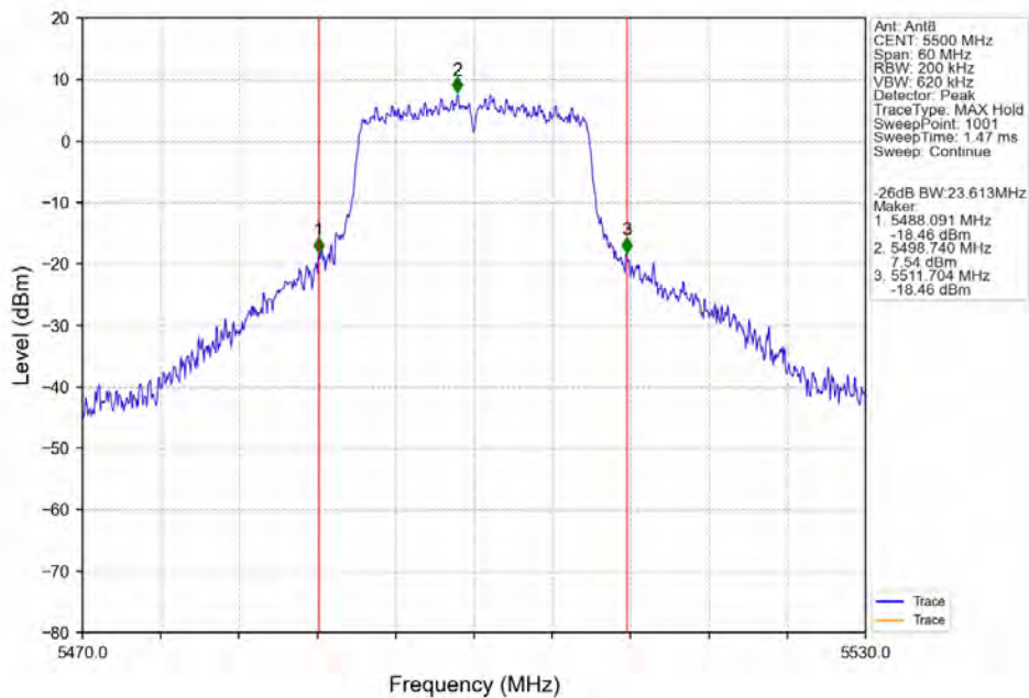
802.11n(HT20)_LCH_5500MHz_Ant8_NTNV
