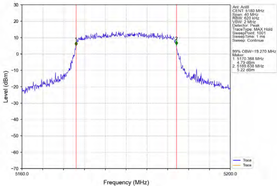
802.11ax(HEW20)_LCH_5180MHz_RU242_Left_Ant8_NTNV
