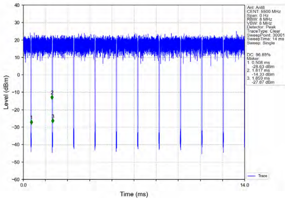
802.11ac(VHT20)_LCH_5500MHz_Ant8_NTNV
