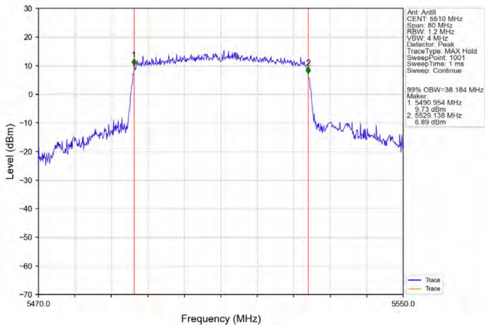
802.11ax(HEW40)_LCH_5510MHz_RU484_Left_Ant8_NTNV
