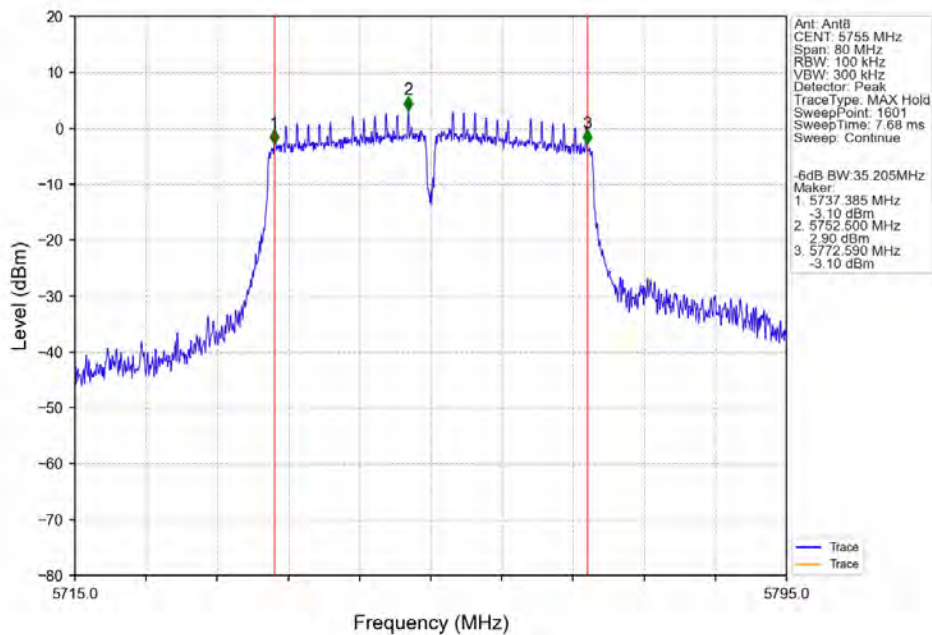
802.11ac(VHT40)_LCH_5755MHz_Ant8_NTNV
