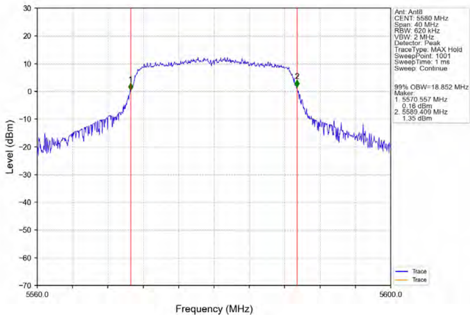
802.11n(HT20)_MCH_5580MHz_Ant8_NTNV
