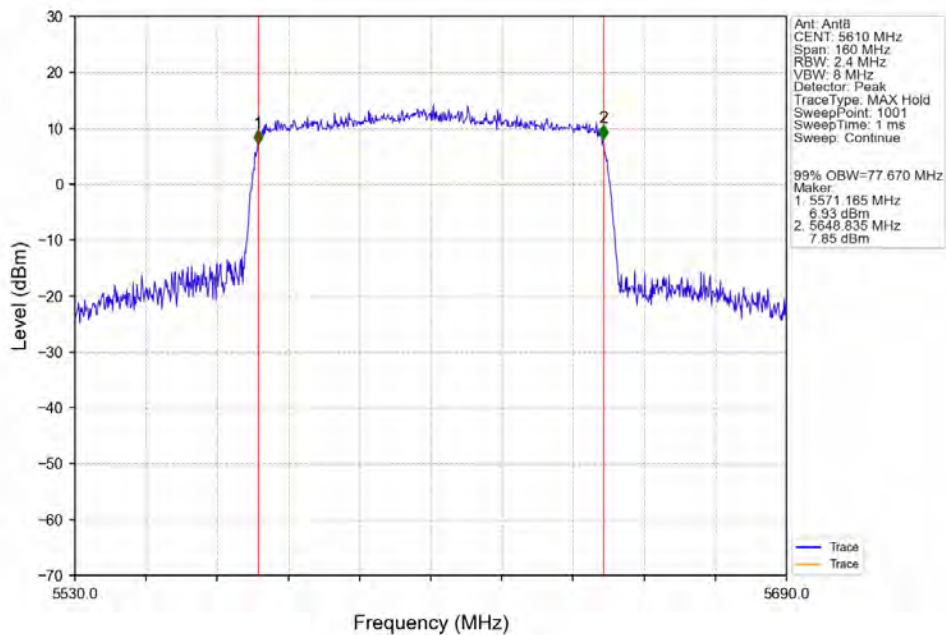
802.11ax(HEW80)_HCH_5610MHz_RU996_Left_Ant8_NTNV
