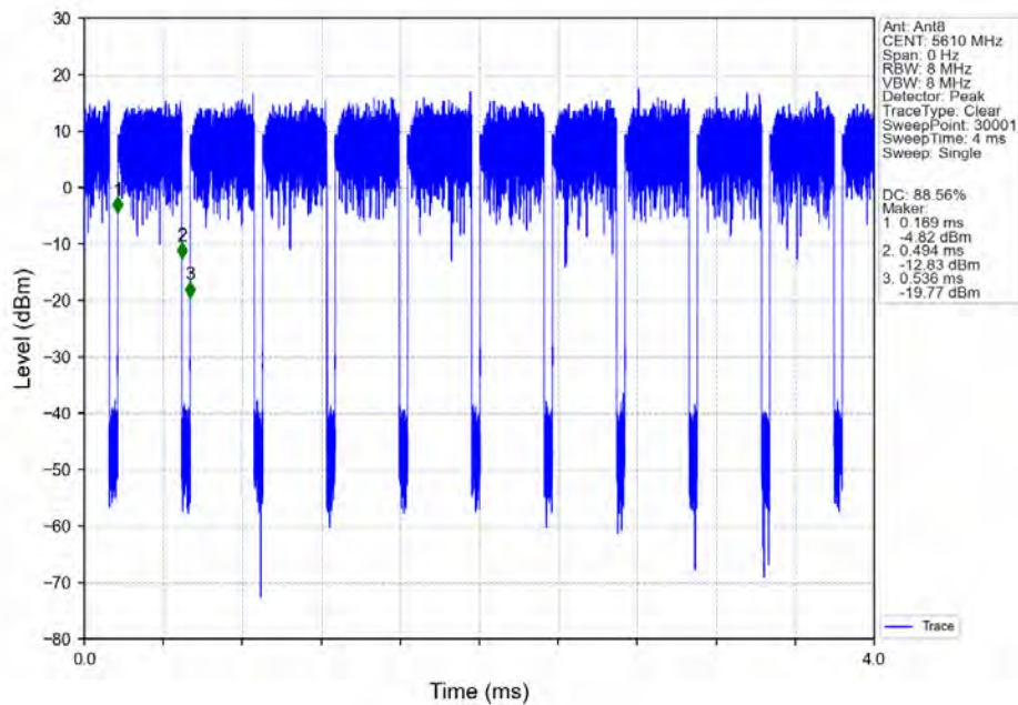
802.11ac(VHT80)_HCH_5610MHz_Ant8_NTNV
