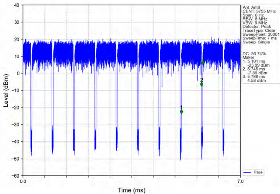
802.11n(HT40)_LCH_5755MHz_Ant8_NTNV
