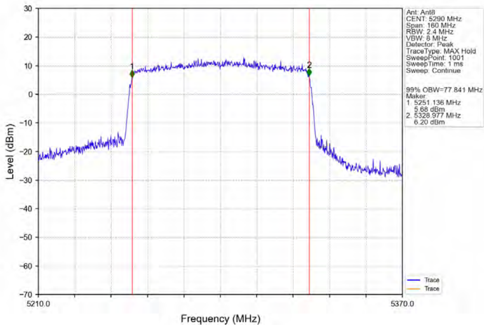
802.11ax(HEW80)_MCH_5290MHz_RU996_Left_Ant8_NTNV
