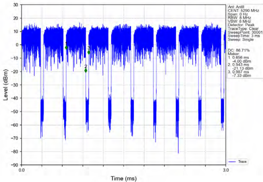
802.11ax(HEW80)_MCH_5290MHz_RU996_Left_Ant8_NTNV
