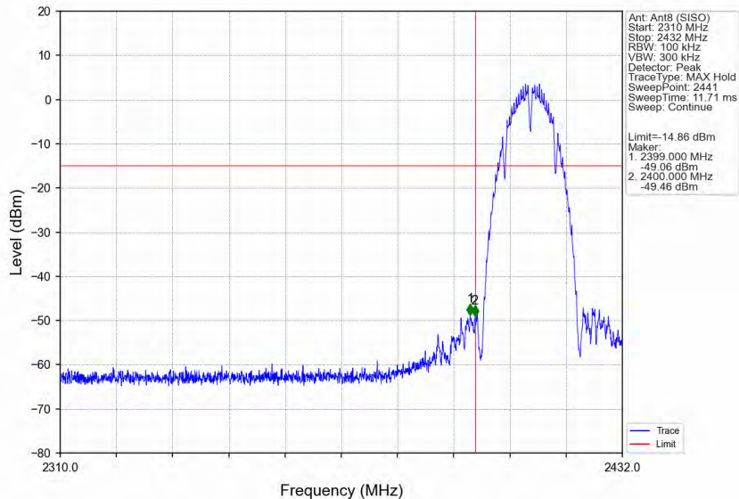
802.11b_LCH_2412MHz_Ant8 (SISO)_NTNV
