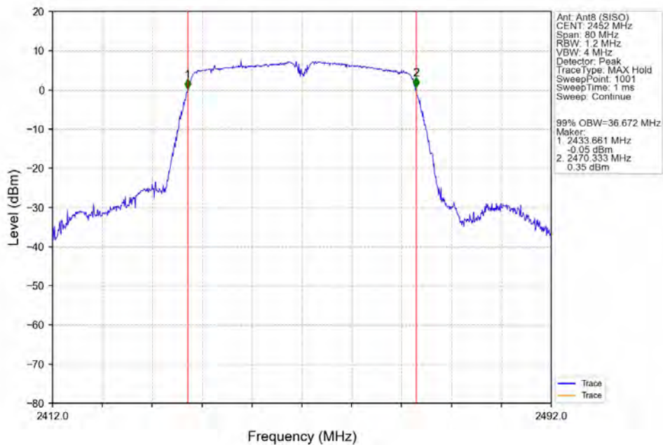
802.11VHT(VHT40)_HCH_2452MHz_Ant8 (SISO)_NTNV
