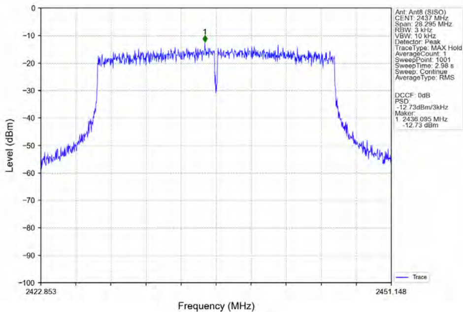
802.11ax(HEW20)_MCH_2437MHz_RU242_Left_Ant8 (SISO)_NTNV
