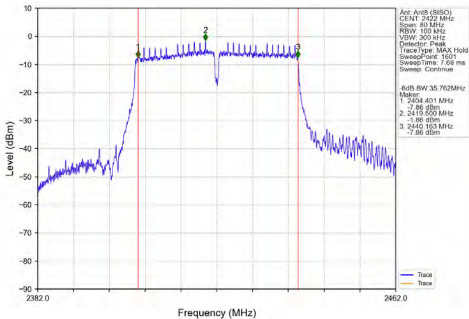
802.11n(HT40)_LCH_2422MHz_Ant8 (SISO)_NTNV
