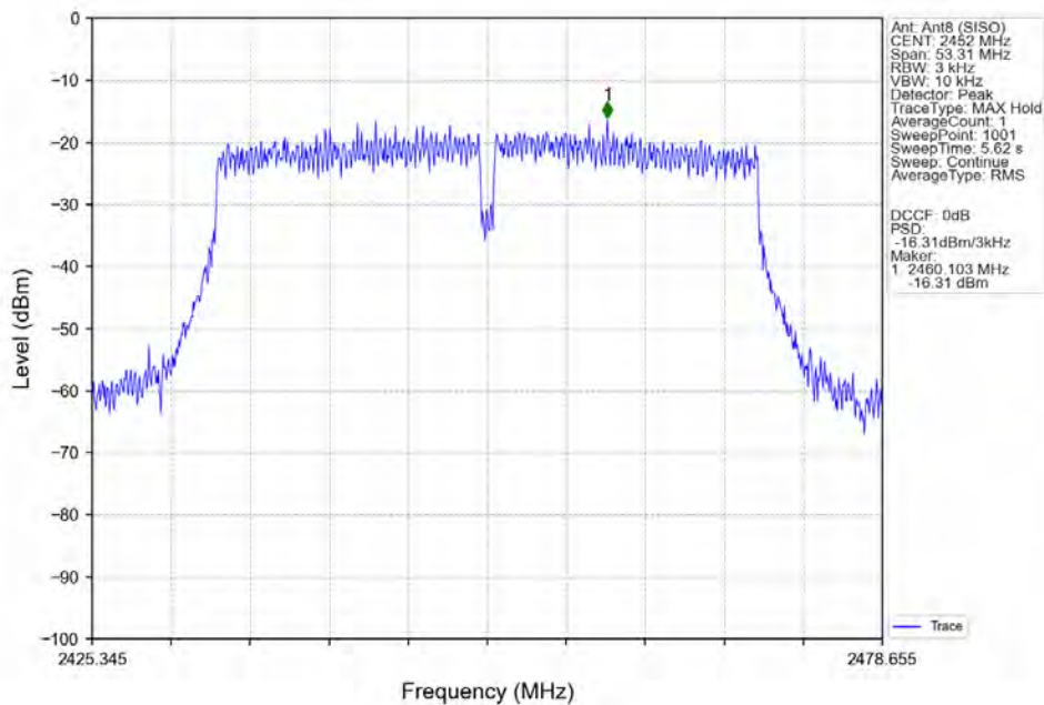
802.11n(HT40)_HCH_2452MHz_Ant8 (SISO)_NTNV
