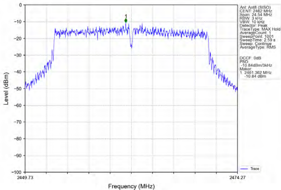
802.11VHT(VHT20)_HCH_2462MHz_Ant8 (SISO)_NTNV
