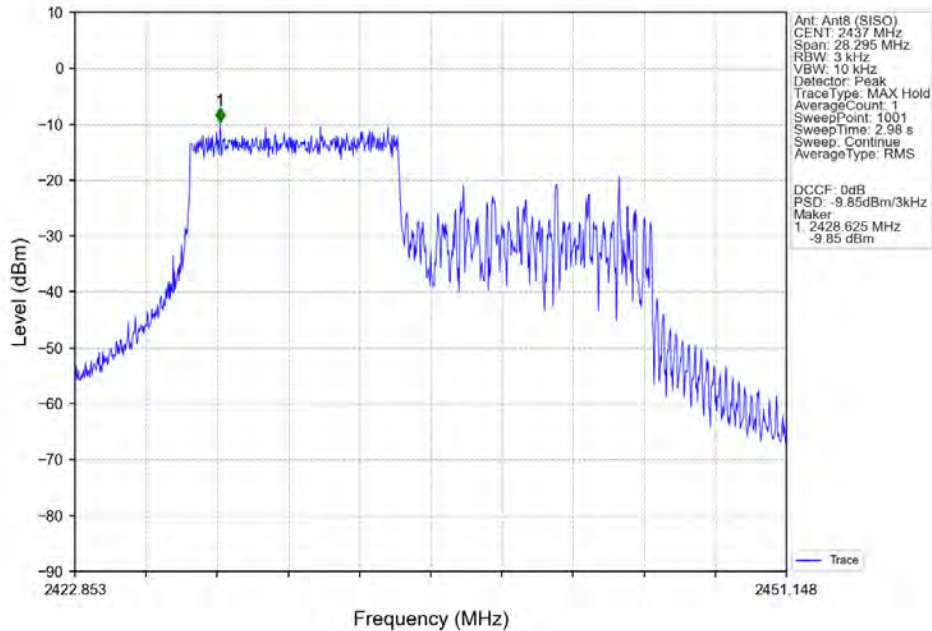
802.11ax(HEW20)_MCH_2437MHz_RU242_Left_Ant8 (SISO)_NTNV
