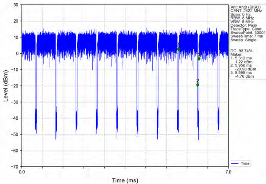
802.11n(HT40)_LCH_2422MHz_Ant8 (SISO)_NTNV
