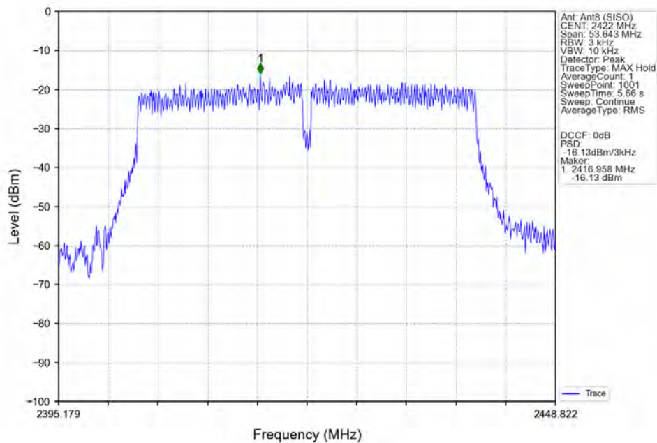
802.11n(HT40)_LCH_2422MHz_Ant8 (SISO)_NTNV
