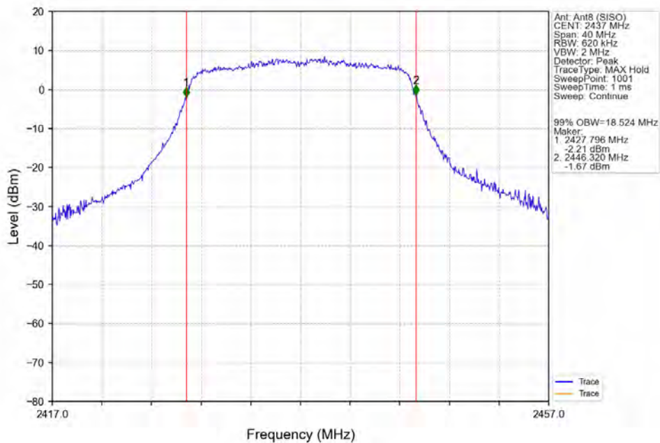
802.11n(HT20)_MCH_2437MHz_Ant8 (SISO)_NTNV
