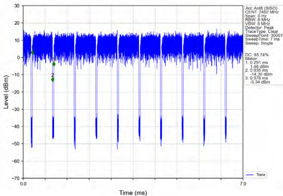
802.11n(HT40)_HCH_2452MHz_Ant8 (SISO)_NTNV
