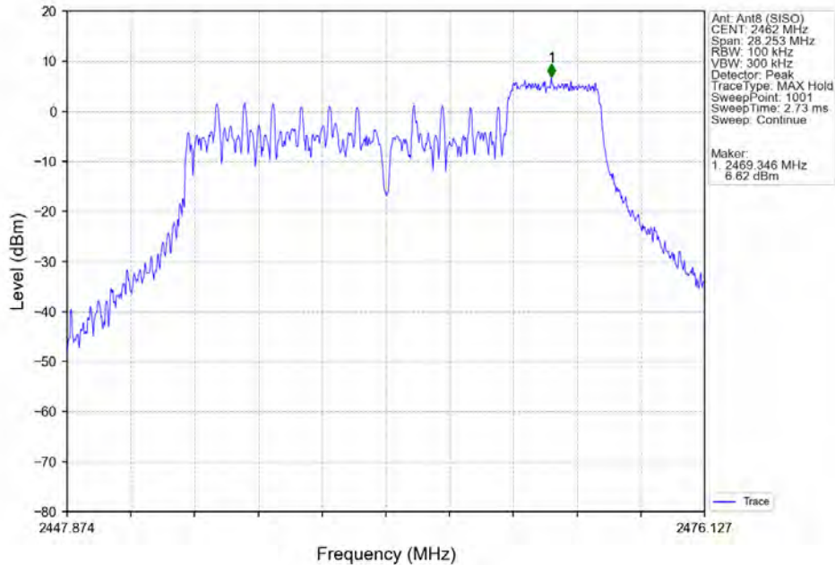
802.11ax(HEW20)_HCH_2462MHz_RU106_Right_Ant8 (SISO)_NTNV
