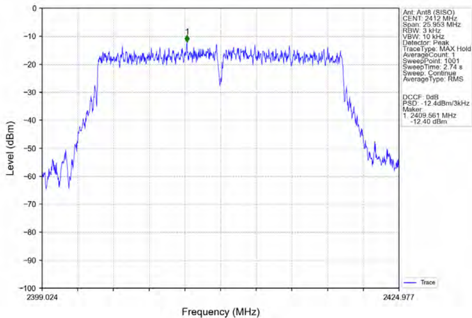
802.11VHT(VHT20)_LCH_2412MHz_Ant8 (SISO)_NTNV
