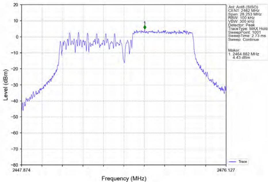
802.11ax(HEW20)_HCH_2462MHz_RU106_Right_Ant8 (SISO)_NTNV
