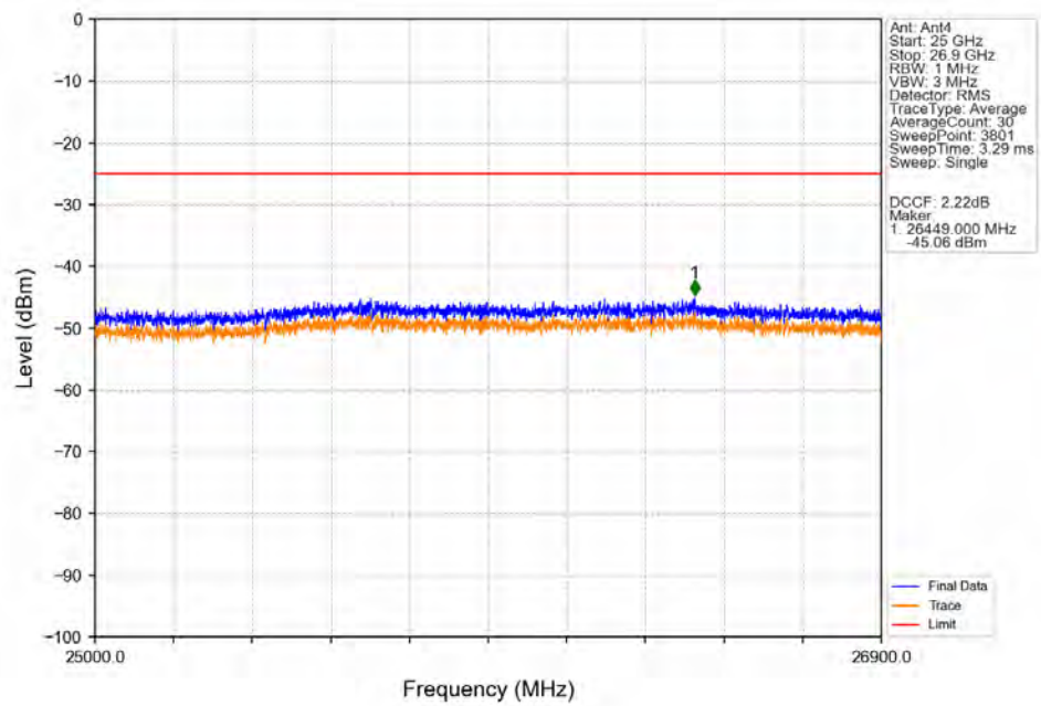
Band41_20MHz_16QAM_MCH_2593MHz_RB_1_0_NTNV
