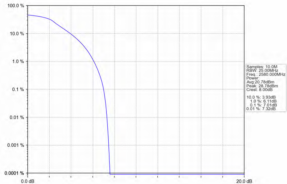
Band38_20MHz_QPSK_LCH_2580MHz_RB_100_0_NTNV
