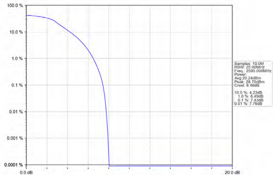
Band38_20MHz_QPSK_MCH_2595MHz_RB_100_0_NTNV
