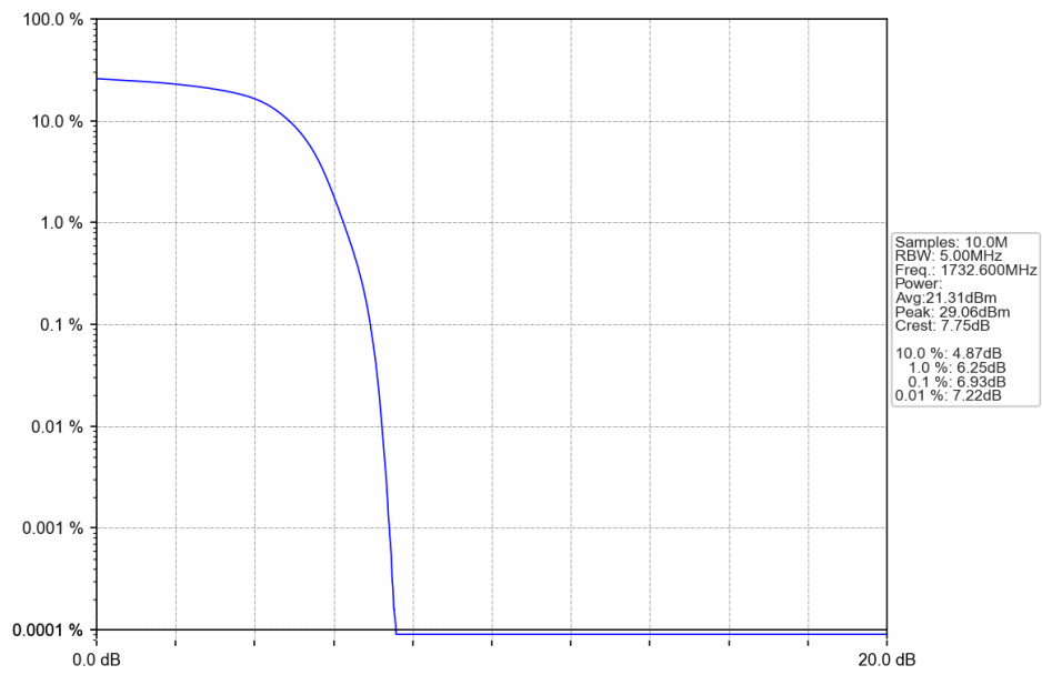
BandIV_HSUPA_MCH_1732.6MHz_Subtest 1_NTNV
