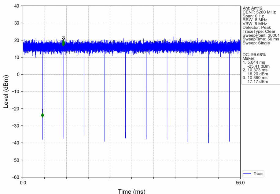
802.11n(HT20)_LCH_5260MHz_Ant12_NTNV
