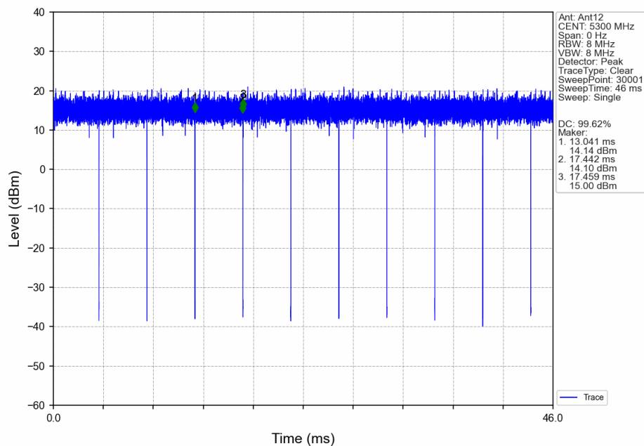
802.11ax(HEW20)_MCH_5300MHz_RU242_Left_Ant12_NTNV
