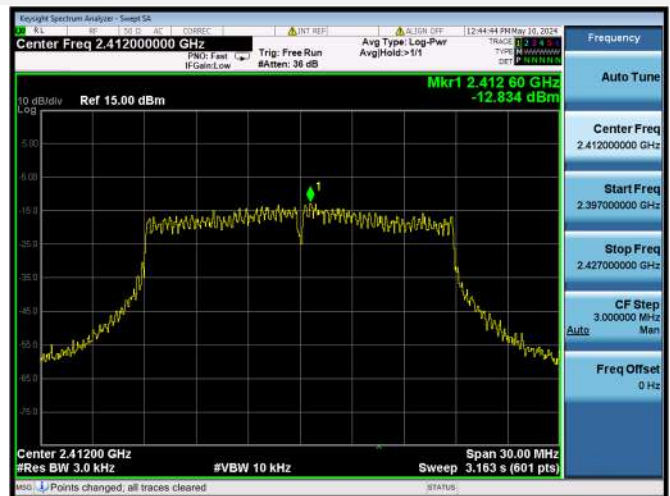
VHT20 CH1
