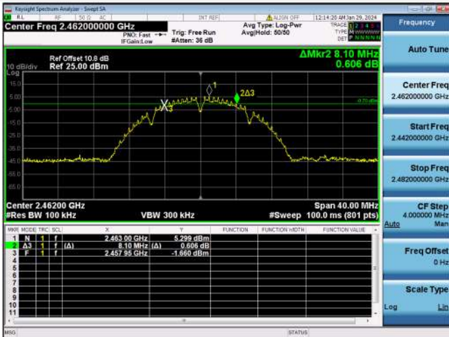
802.11b CH11
