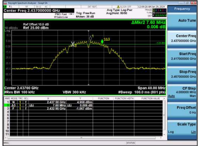
802.11b CH6
