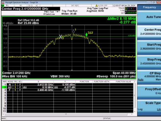
802.11b CH1
