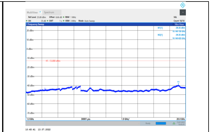
GSM1900-661-0-1000~20000MHz
