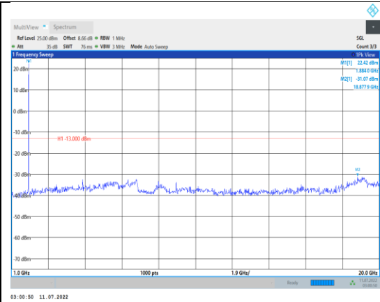
Band2-3MHz-QPSK-18900-1RB#0- Range2:1000~20000MHz
