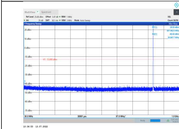
GPRS850-190-3-30~1000MHz
