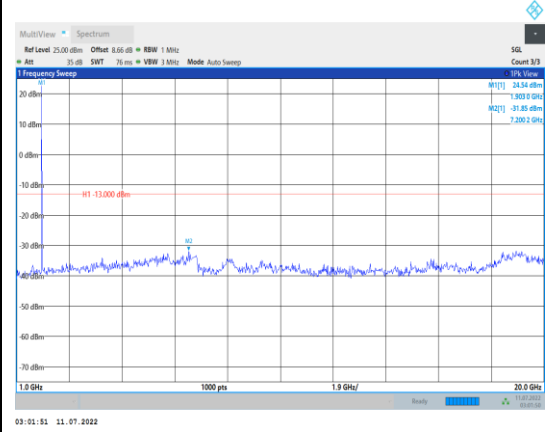
Band2-3MHz-QPSK-19185-1RB#0- Range2:1000~20000MHz
