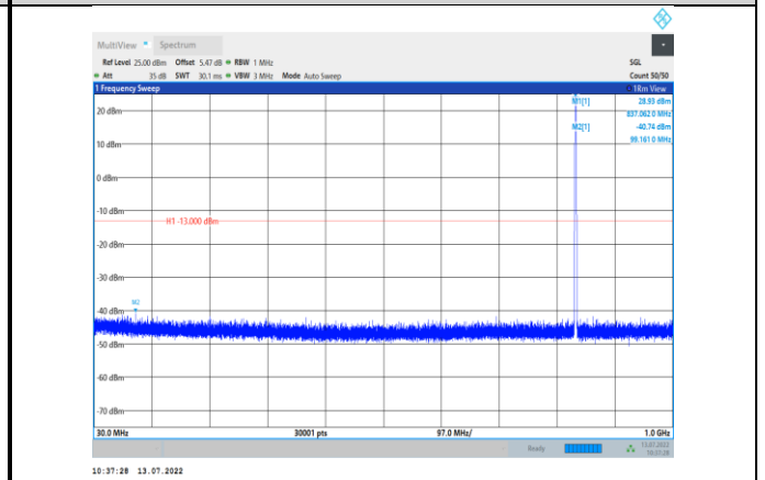
GPRS850-251-3-30~1000MHz
