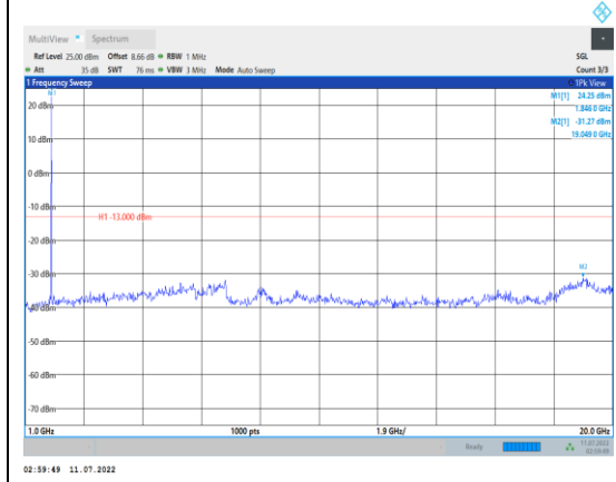
Band2-3MHz-QPSK-18615-1RB#0- Range2:1000~20000MHz
