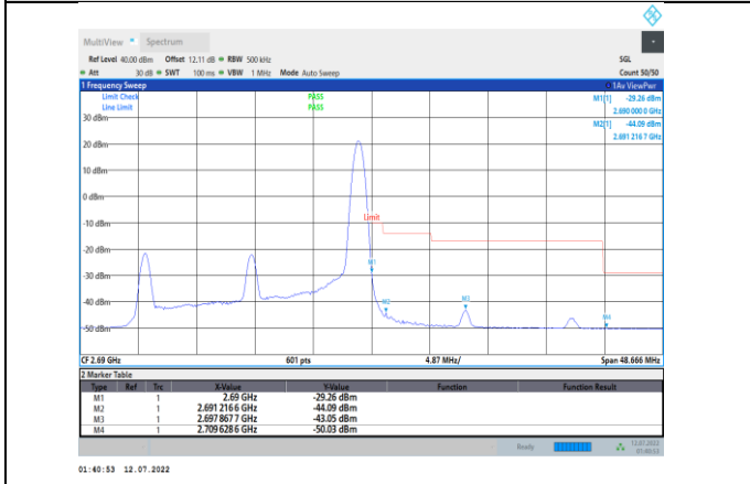
Band41-20MHz-16QAM-41490-1RB#99
