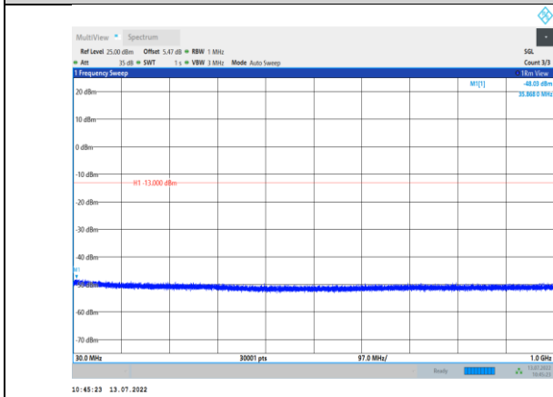
GSM1900-661-0-30~1000MHz
