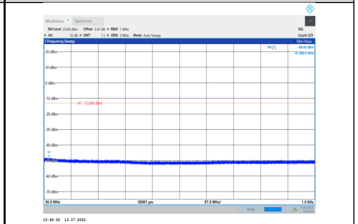
GSM1900-810-0-30~1000MHz
