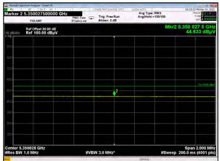
U-NII-2A 11ac20 CH64 AV
