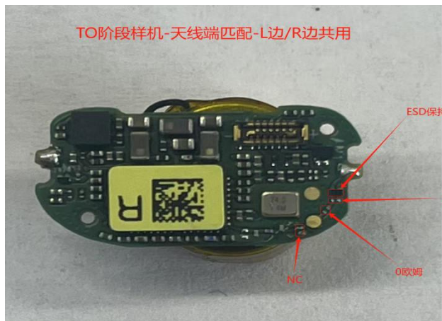
L边/R边主板天线端匹配:
