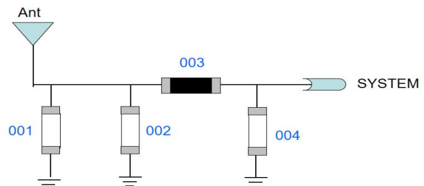
L边/R边主板天线端匹配:
