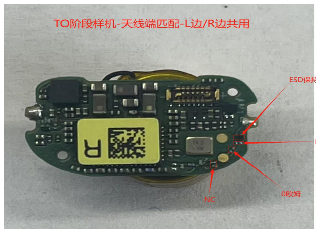
L边/R边主板天线端匹配:
