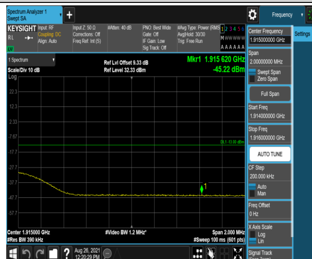
Band25-20MHz-16QAM-26590-1RB#99
