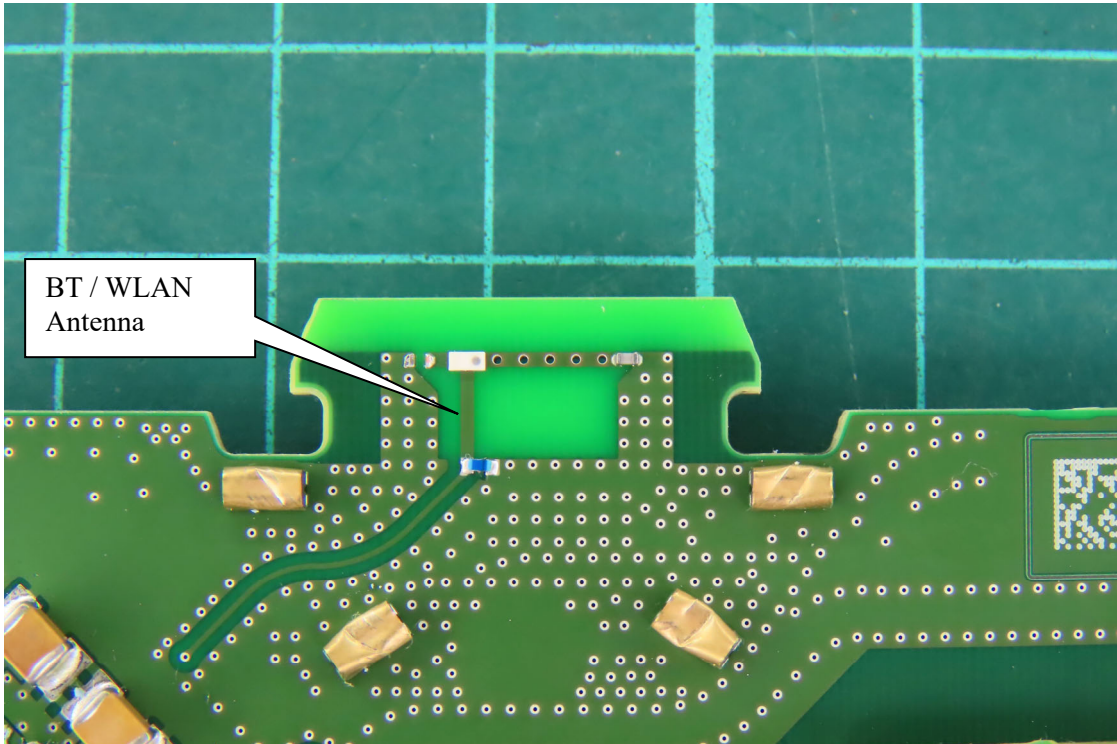
(19) EUT Photo
