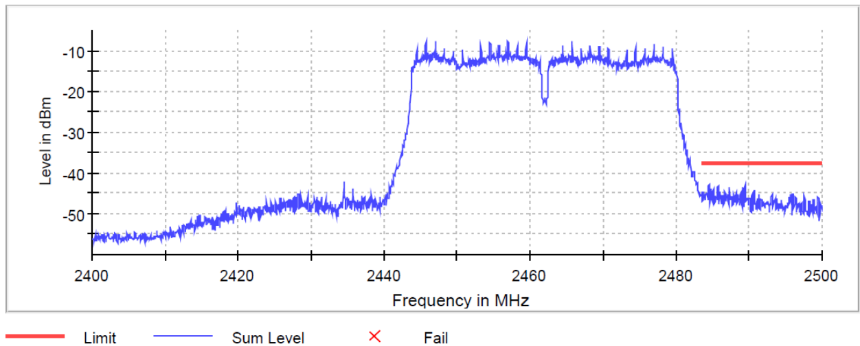
Band Edge
