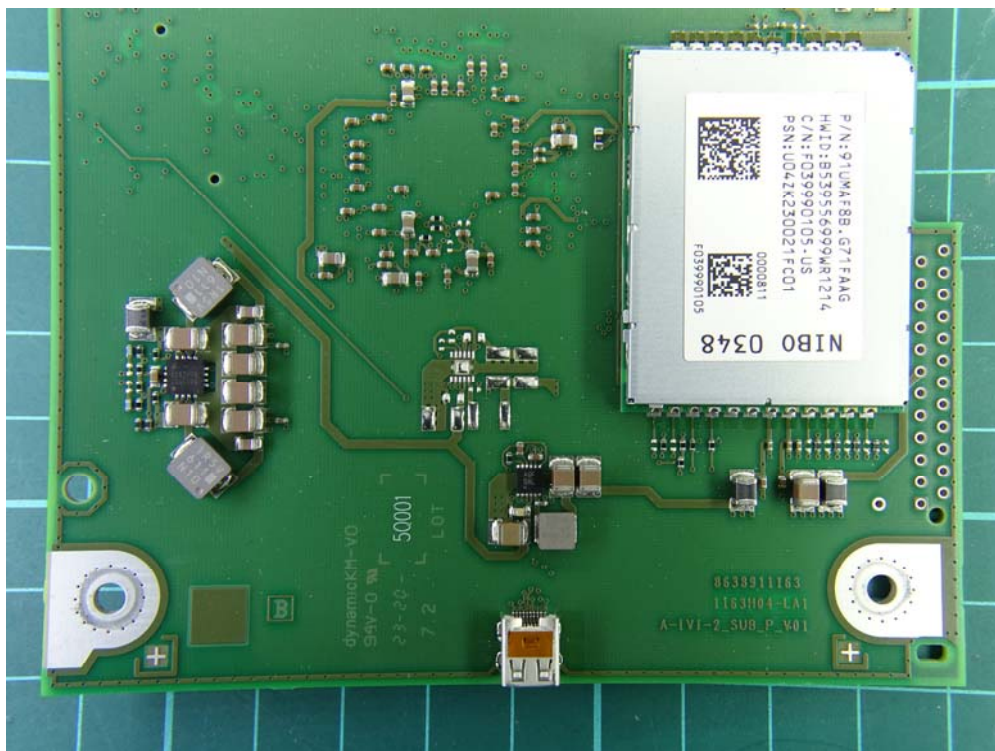
(56) EUT Photo
