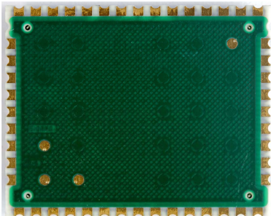
(28) EUT Photo (RF Module)
