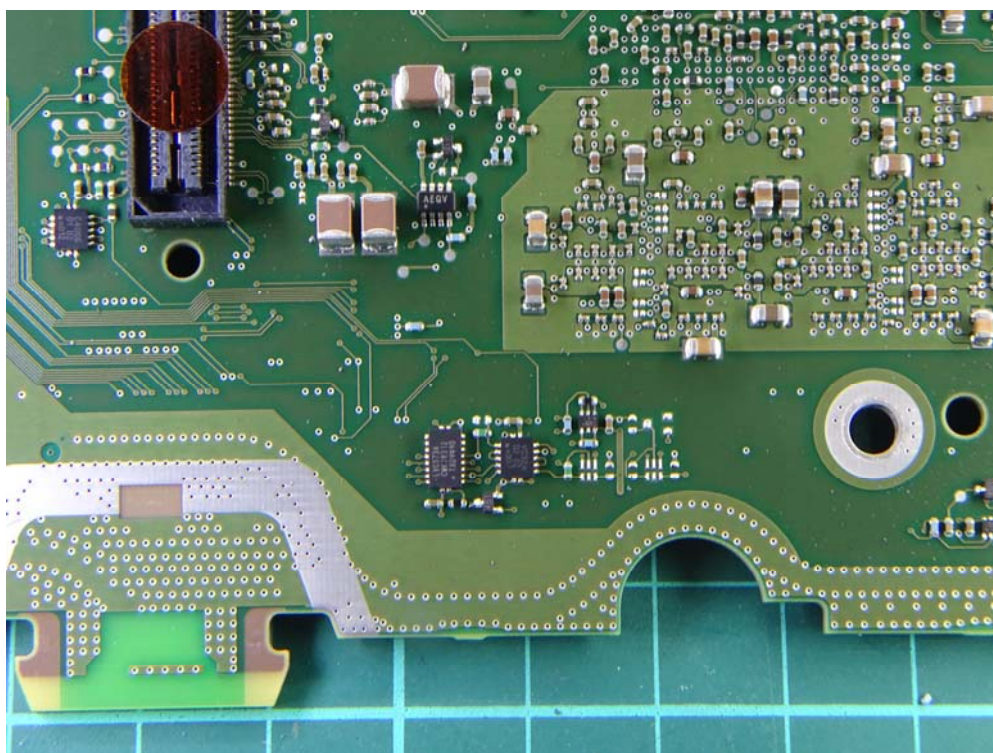
(40) EUT Photo
