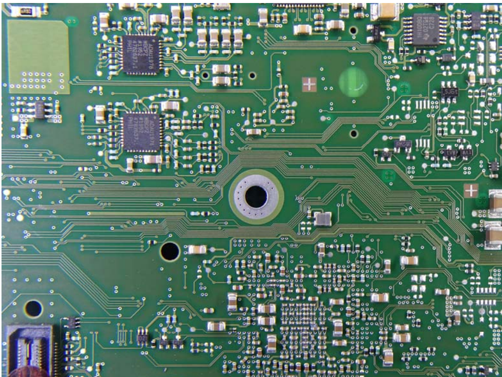
(36) EUT Photo
