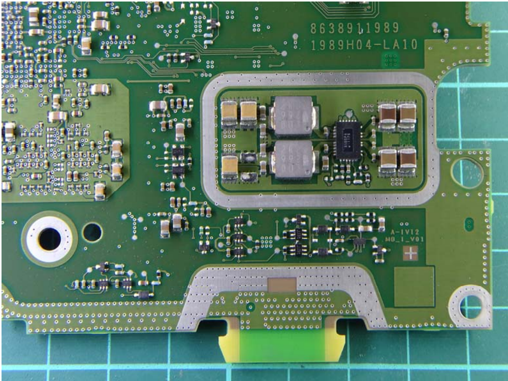
(41) EUT Photo
