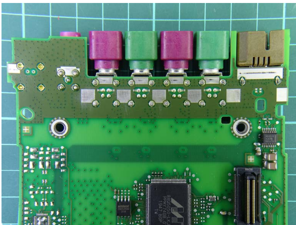
(46) EUT Photo
