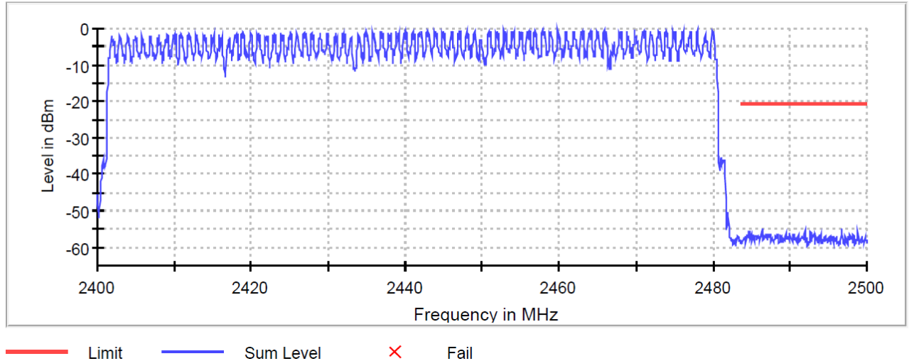
Band Edge
