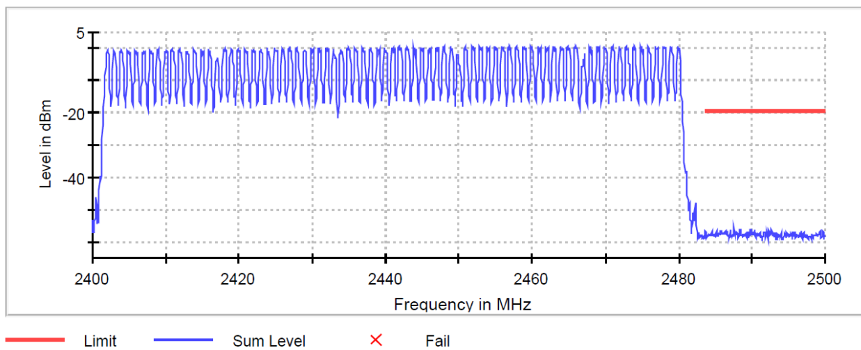
Band Edge
