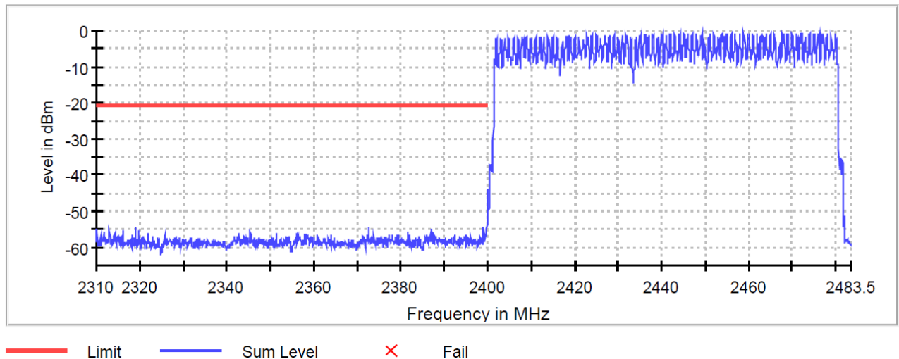
Band Edge
