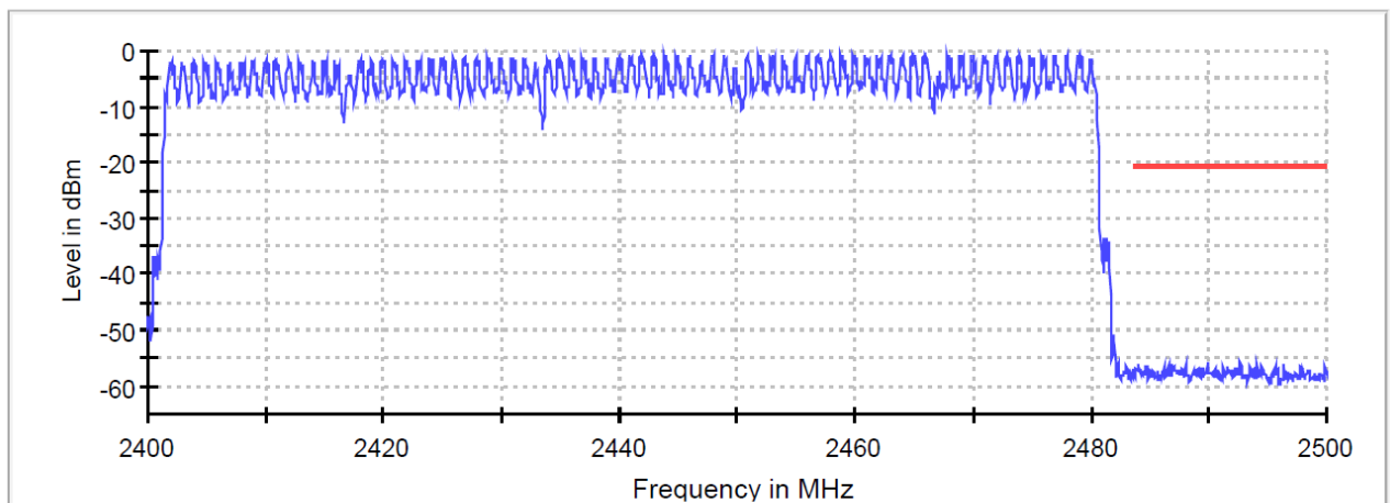
Band Edge
