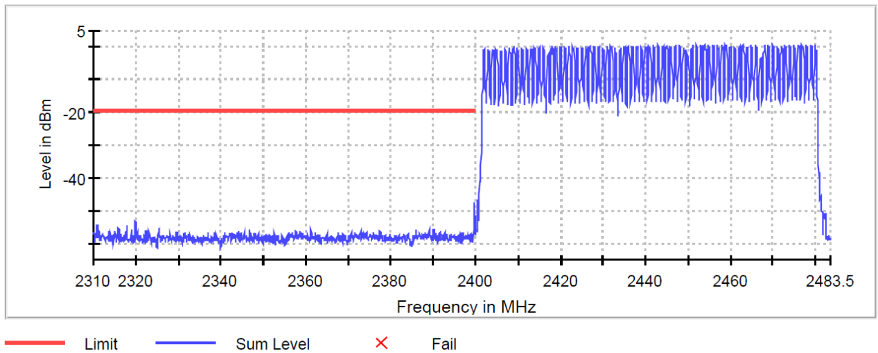
Band Edge
