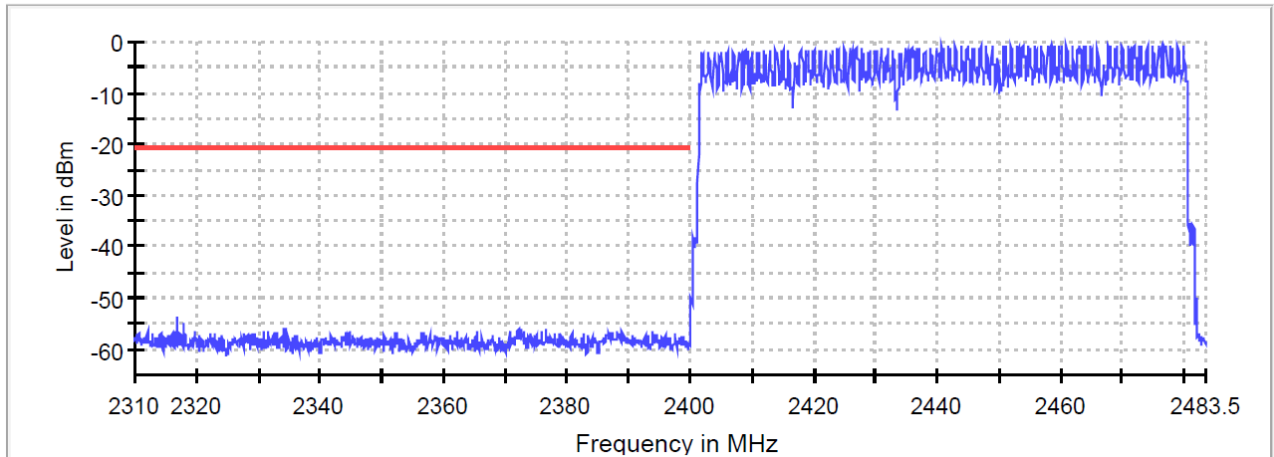
Band Edge
