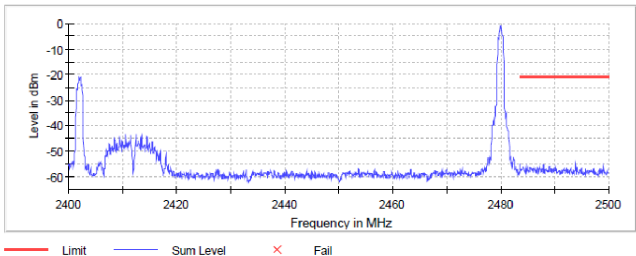
Band Edge
