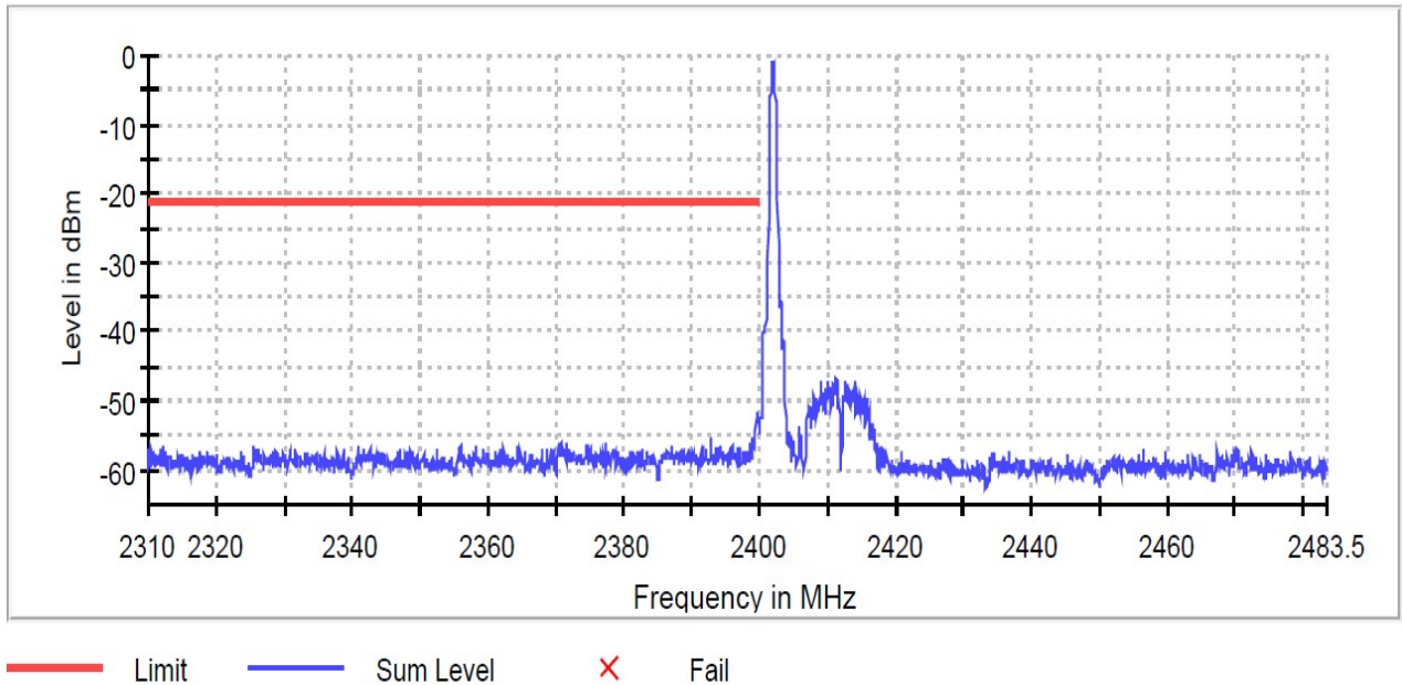
Band Edge
