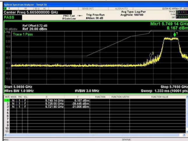
802.11(n40)-5755
