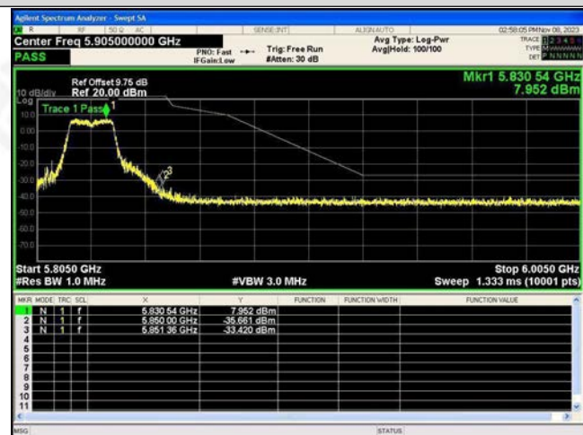
802.11(n20)-5825
