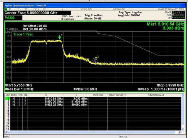
802.11ac(VH20)-5825
