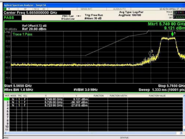
802.11(n20)-5745
