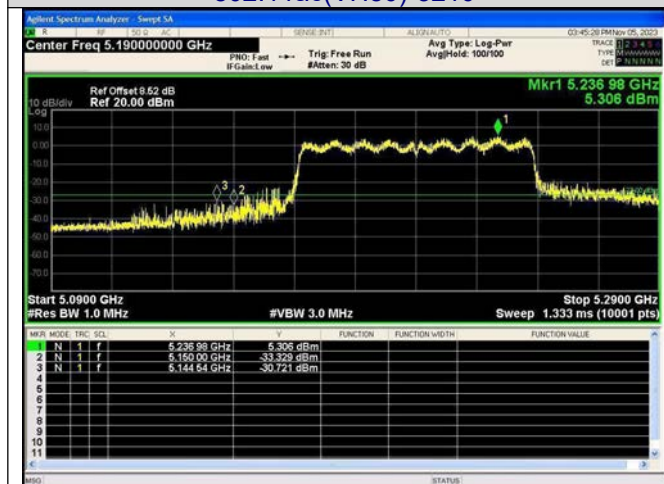
802.11ac(VH80)-5210
