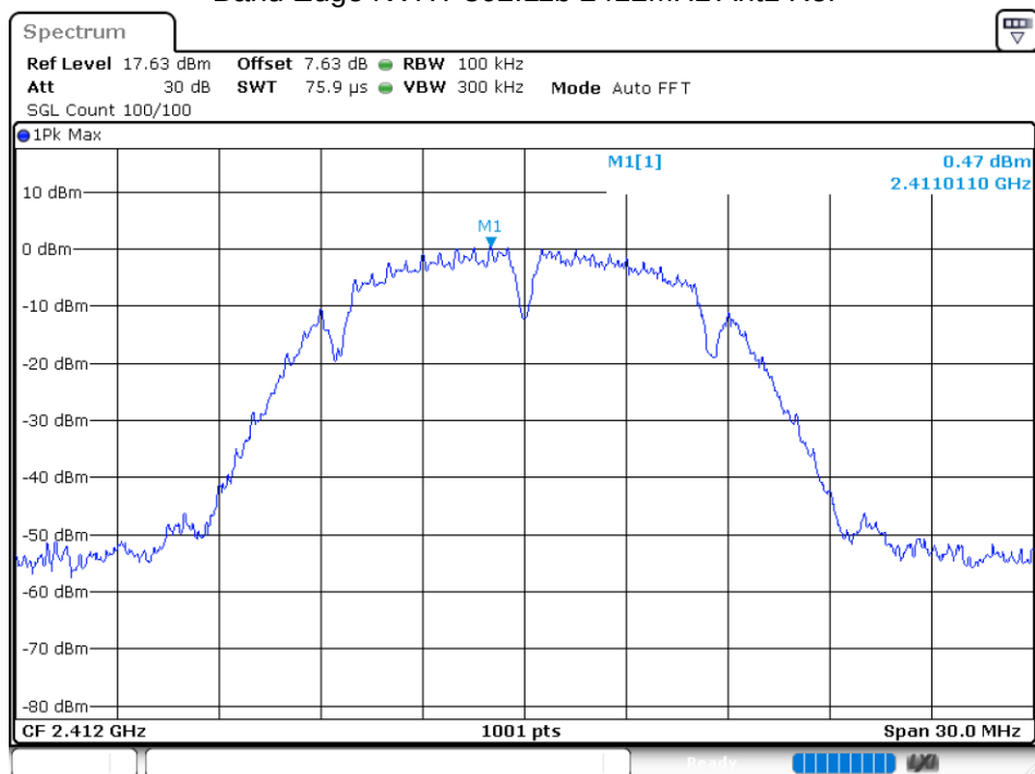
Band Edge NVHT 802.11b 2412MHz Ant1 Ref
