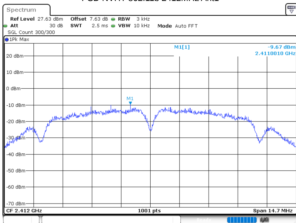
PSD NVHT 802.11b 2412MHz Ant1
