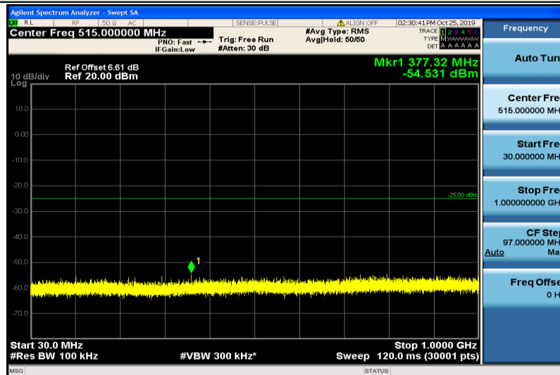
Band7-10MHz-QPSK-20800-1RB#0-30~1000MHz
