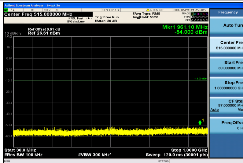
Band2-5MHz-QPSK-18625-1RB#0-30~1000MHz
