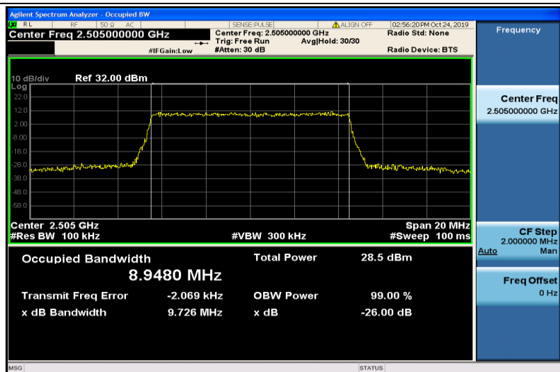
Band7-10MHz-QPSK-20800-50RB#0-8.9480
