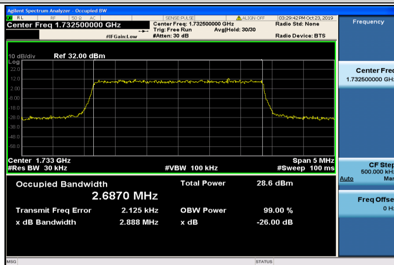
Band4-3MHz-QPSK-20175-15RB#0-2.6870
