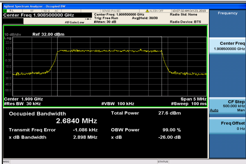
Band2-3MHz-QPSK-19185-15RB#0-2.6840
