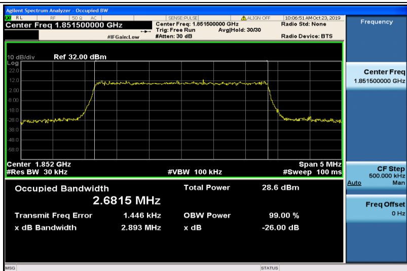
Band2-3MHz-QPSK-18615-15RB#0-2.6815
