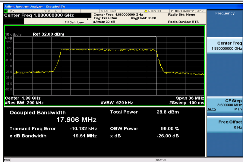
Band2-20MHz-QPSK-18900-100RB#0-17.906
