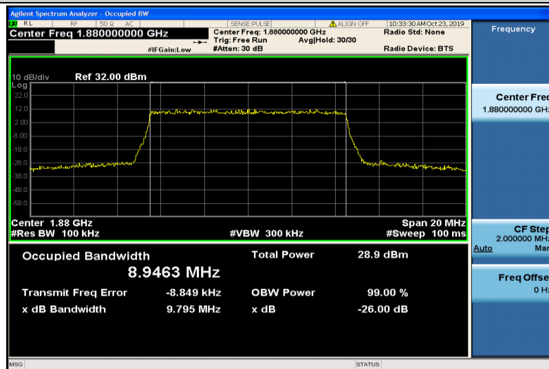
Band2-10MHz-QPSK-18900-50RB#0-8.9463
