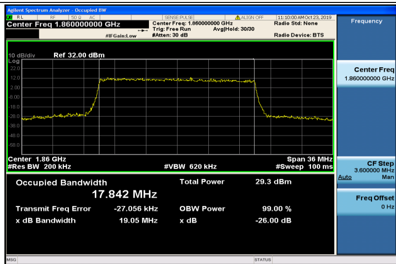
Band2-20MHz-QPSK-18700-100RB#0-17.842
