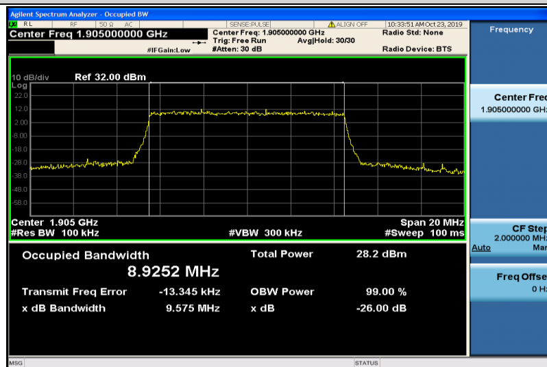
Band2-10MHz-QPSK-19150-50RB#0-8.9252
