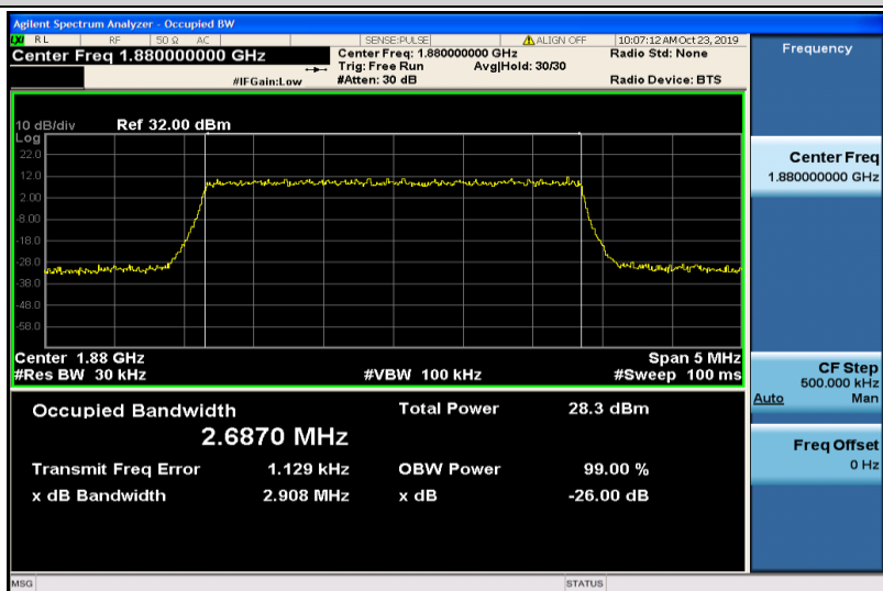
Band2-3MHz-QPSK-18900-15RB#0-2.6870
