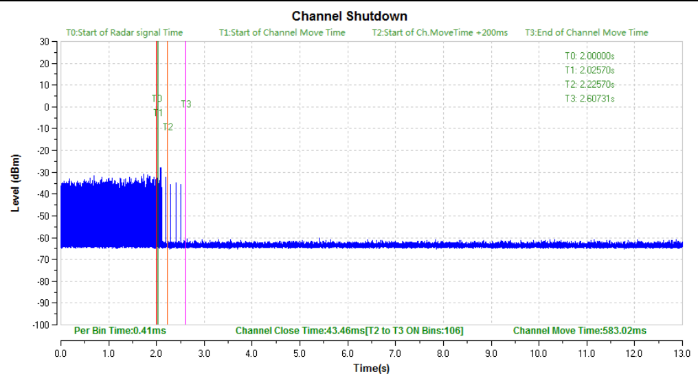
40MHz/5270MHz
