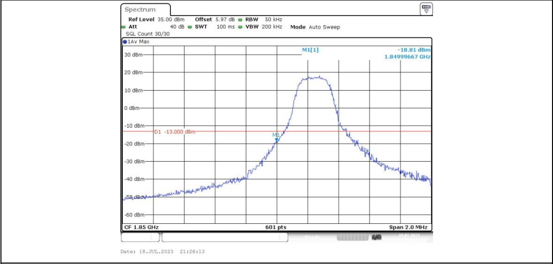
Band2-3MHz-QPSK-18615-1RB#14
