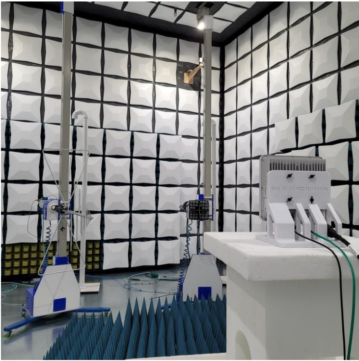
Setup 4. Test Setup 1-18GHz - SU
