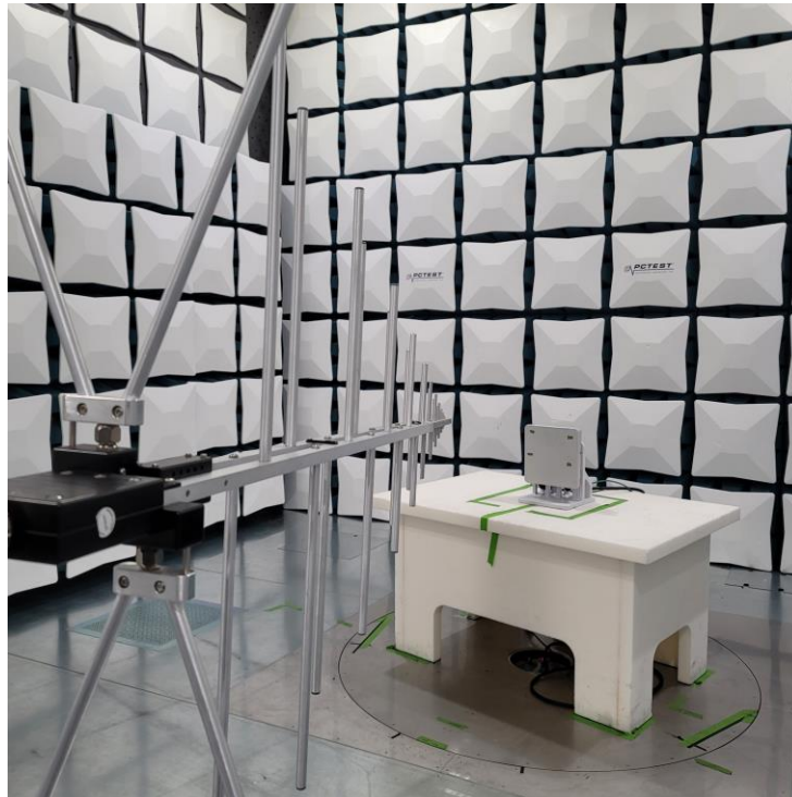
Setup 1. Test Setup <1GHz – SU
