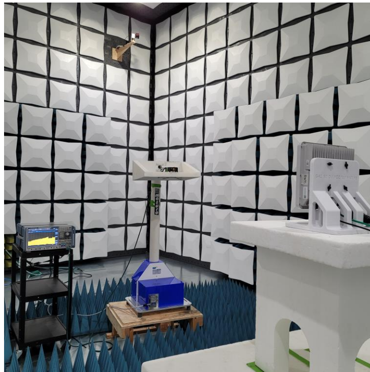
Setup 8. Test Setup >40GHz - SU
