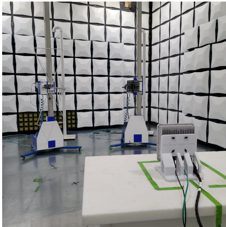
Setup 2. Test Setup <1GHz - SU
