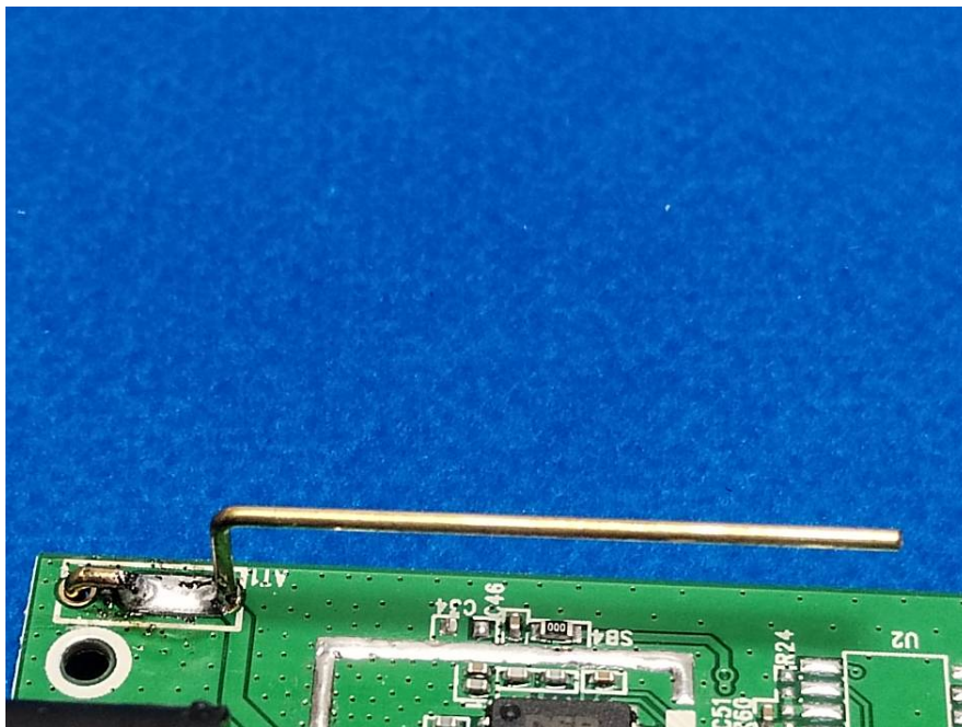
FP Antenna
