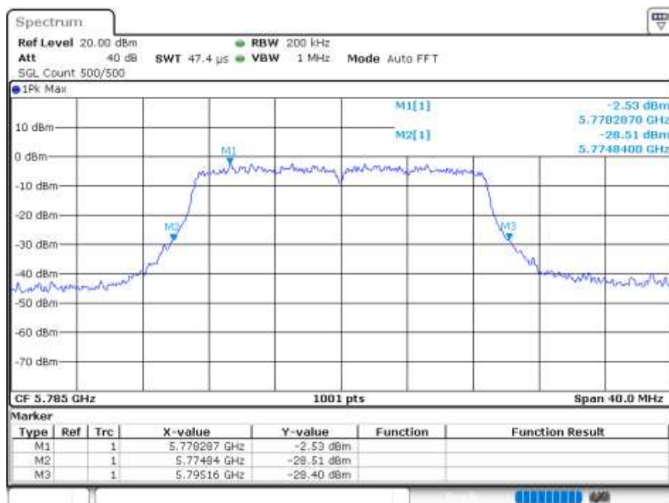
-26 dB BW NVNT 802.11n(HT20) 5785MHz Ant 0
