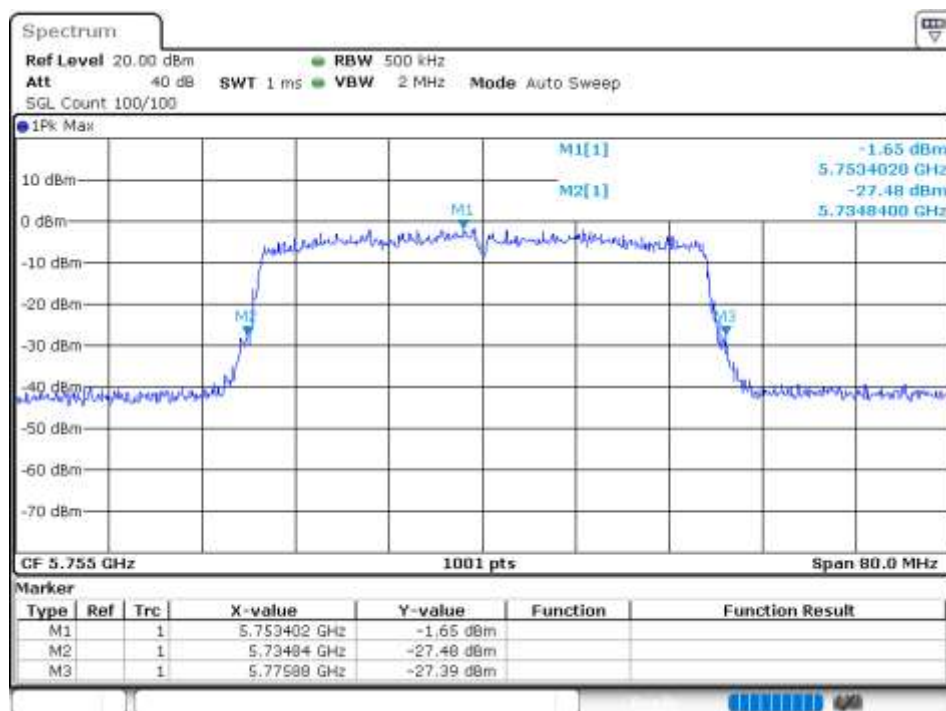
-26 dB BW NVNT 802.11ax40 5755MHz Ant 0
