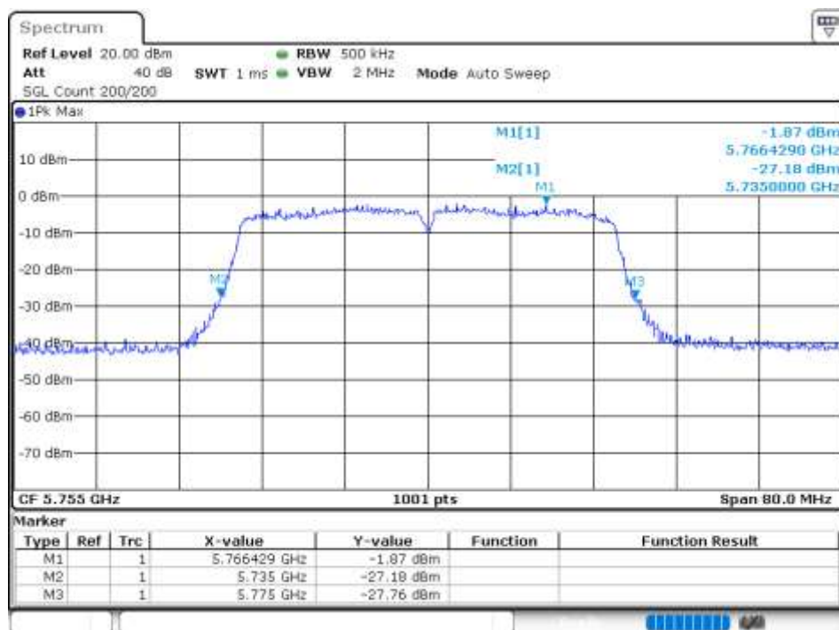
-26 dB BW NVNT 802.11ac40 5755MHz Ant 0
