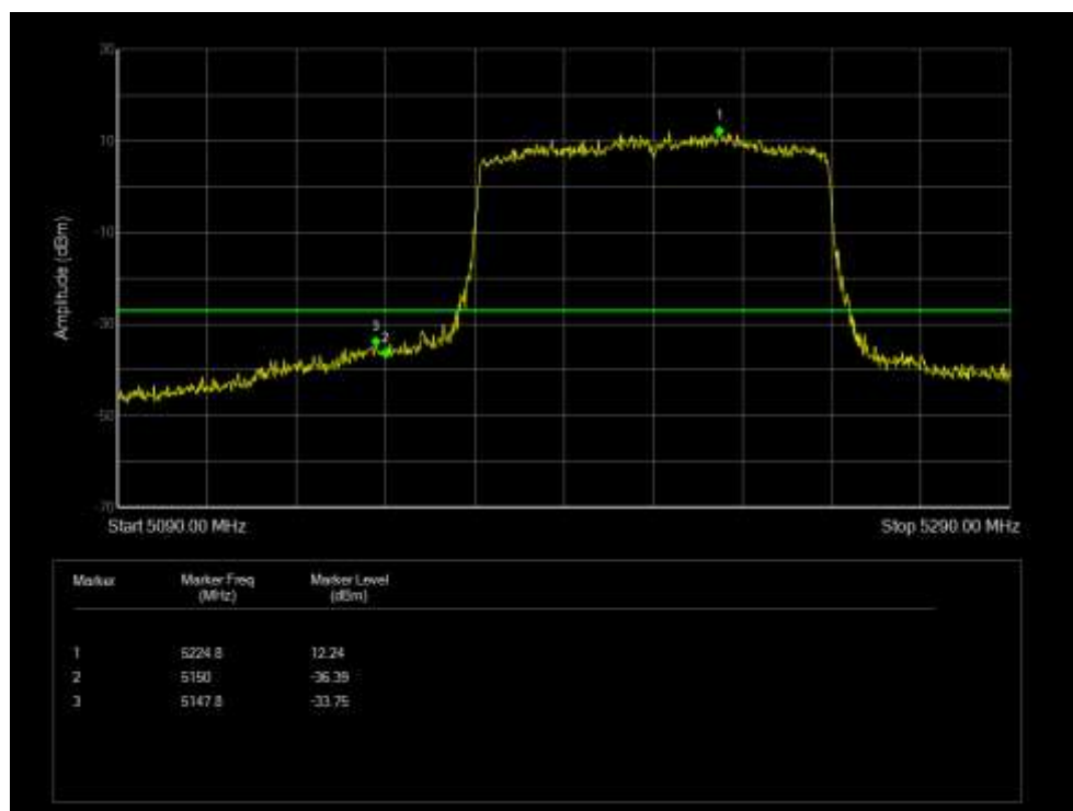
Band Edge NVNT 802.11ax80 5210MHz High Ant 6
