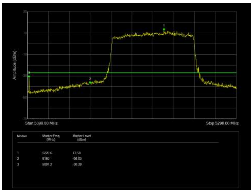
Band Edge NVNT 802.11ax80 5210MHz High Ant 5
