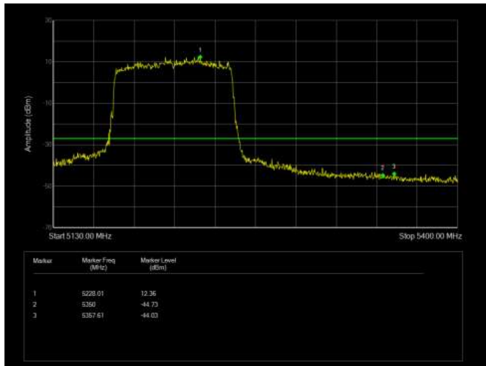
Band Edge NVNT 802.11ax80 5210MHz Low Ant 5
