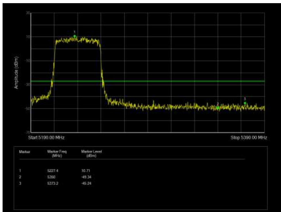
Band Edge NVNT 802.11ax80 5210MHz High Ant 4
