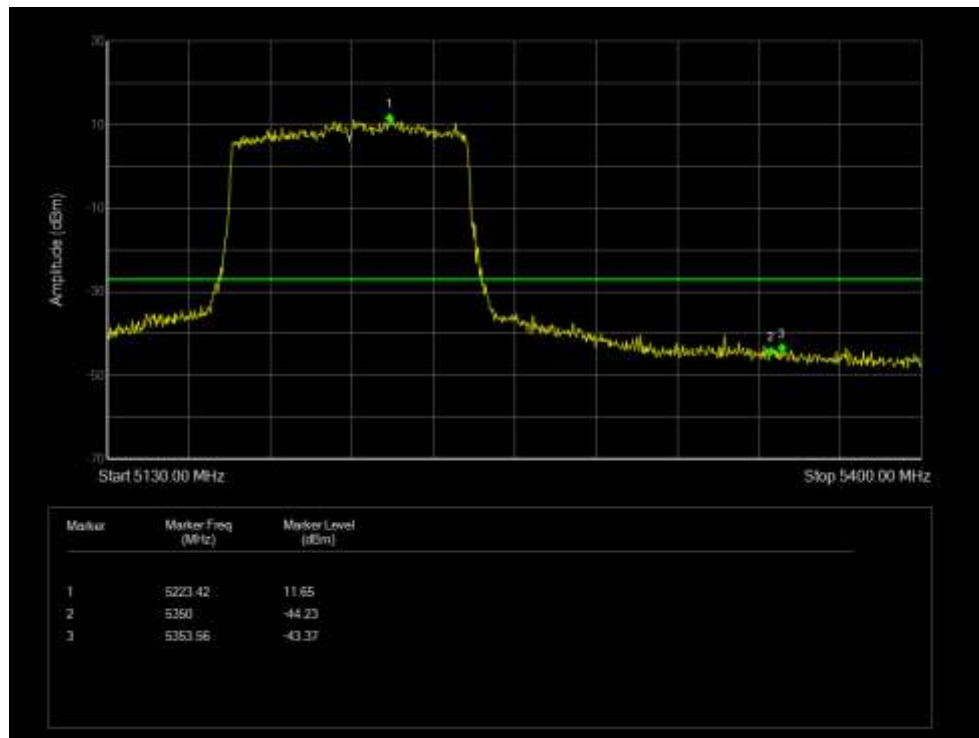
Band Edge NVNT 802.11ax80 5210MHz Low Ant 4
