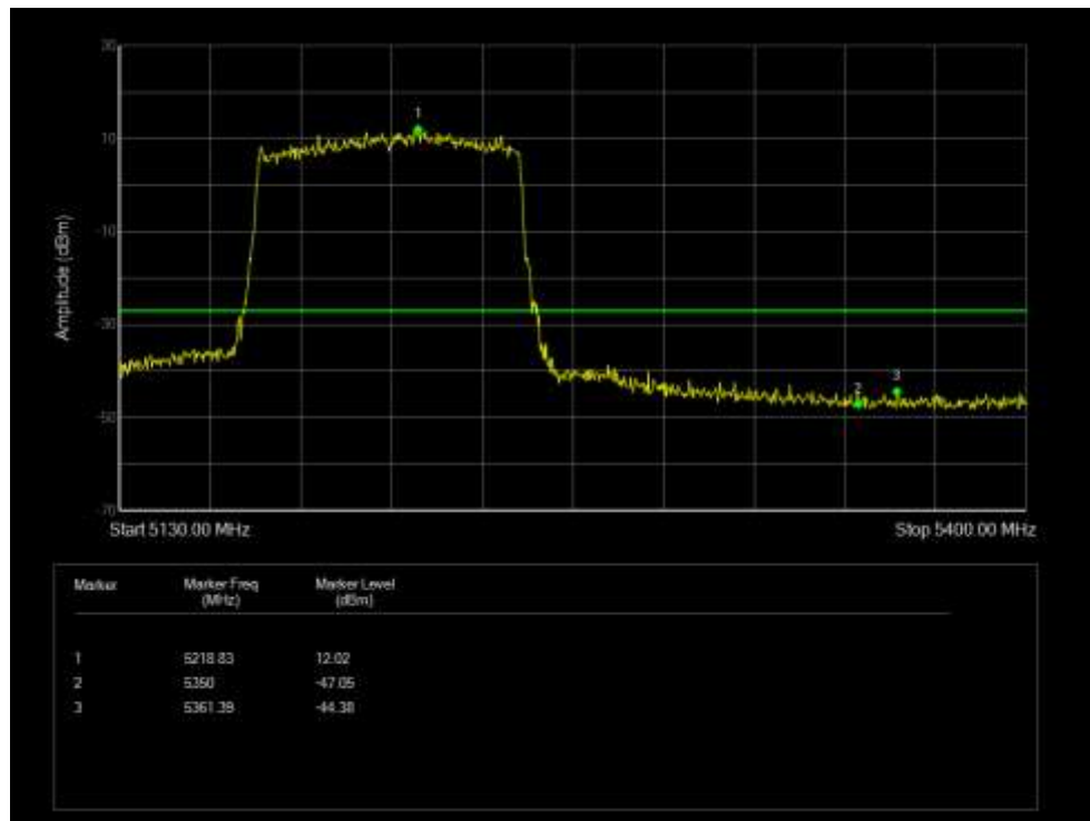
Band Edge NVNT 802.11ax80 5210MHz Low Ant 7
