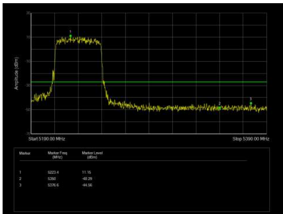
Band Edge NVNT 802.11ax40 5190MHz Low Ant 6
