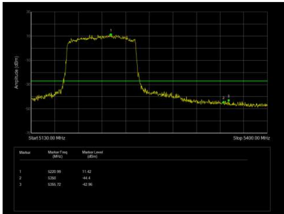
Band Edge NVNT 802.11ax80 5210MHz Low Ant 6
