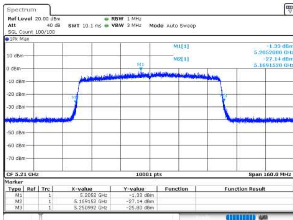
-26 dB BW NVNT 802.11ax80 5210MHz Ant 7
