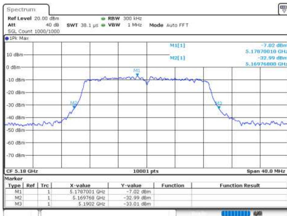
-26 dB BW NVNT 802.11n(HT20) 5180MHz Ant 5
