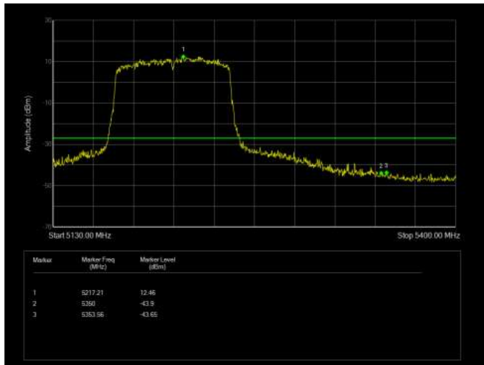
Band Edge NVNT 802.11ac80 5210MHz Low Ant 6
