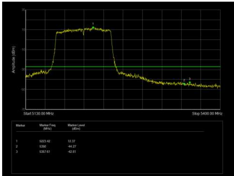
Band Edge NVNT 802.11ac80 5210MHz Low Ant 4
