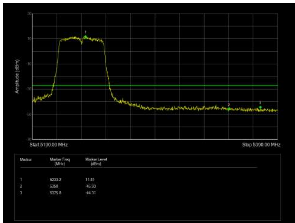
Band Edge NVNT 802.11ac40 5190MHz Low Ant 7
