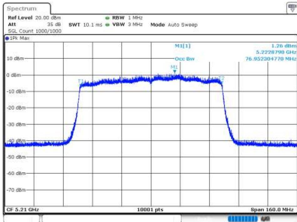
-26 dB BW NVNT 802.11ax80 5210MHz Ant 4
