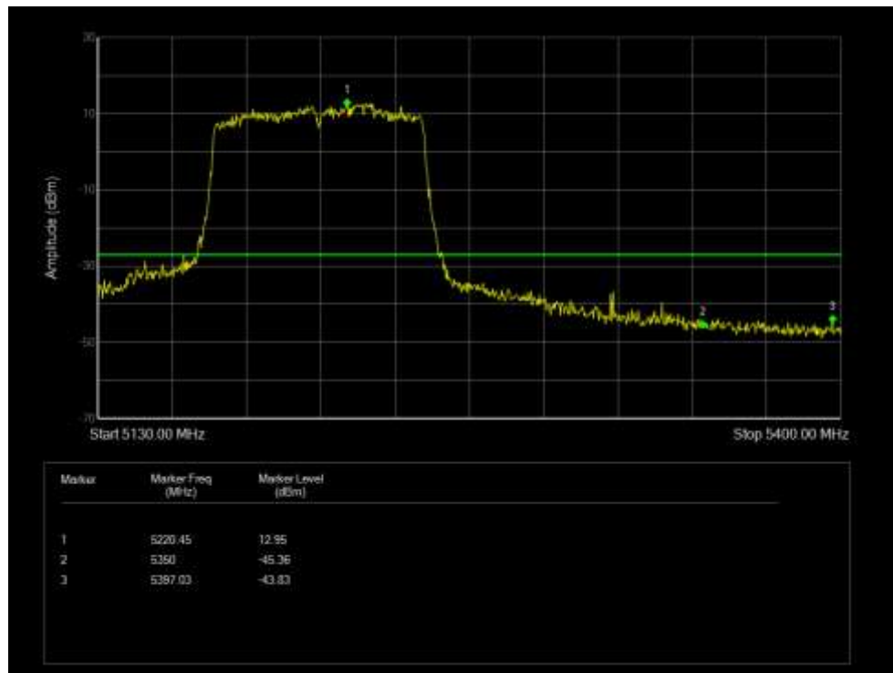
Band Edge NVNT 802.11ac80 5210MHz Low Ant 5
