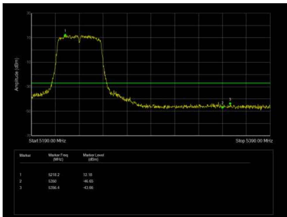
Band Edge NVNT 802.11ac40 5190MHz Low Ant 5
