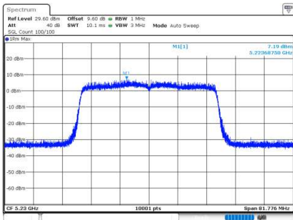
PSD NVNT 802.11ax40 5230MHz Ant 4
