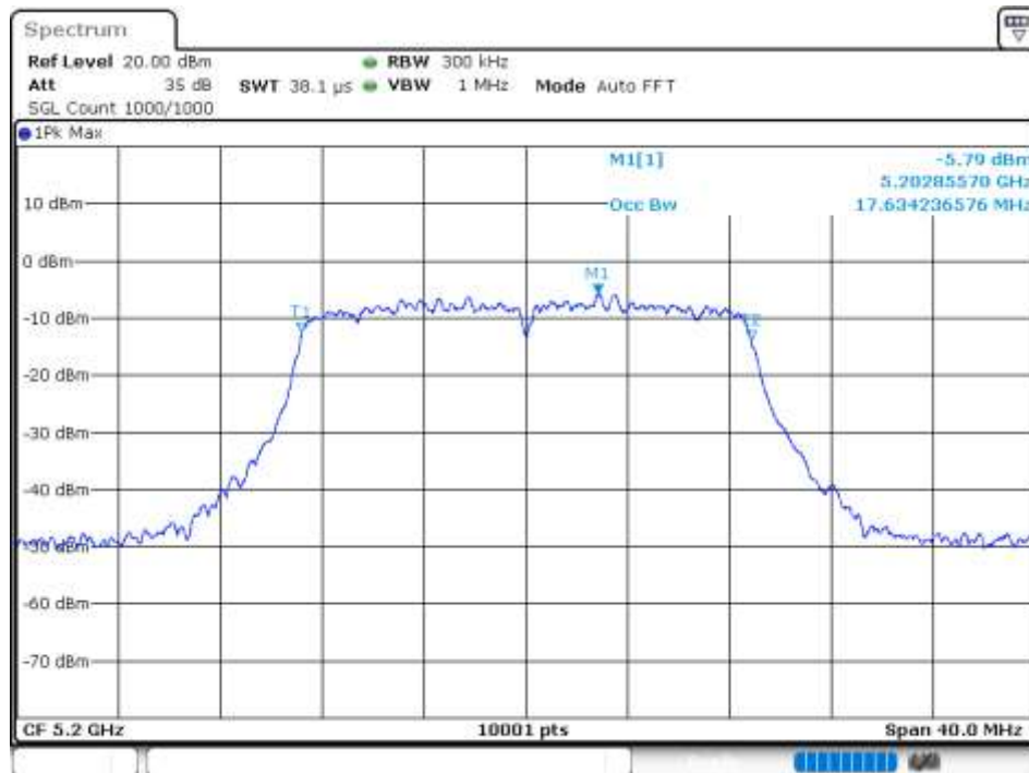
-26 dB BW NVNT 802.11n(HT20) 5200MHz Ant 6
