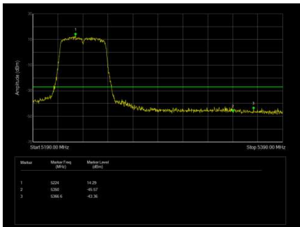
Band Edge NVNT 802.11ac40 5190MHz Low Ant 6
