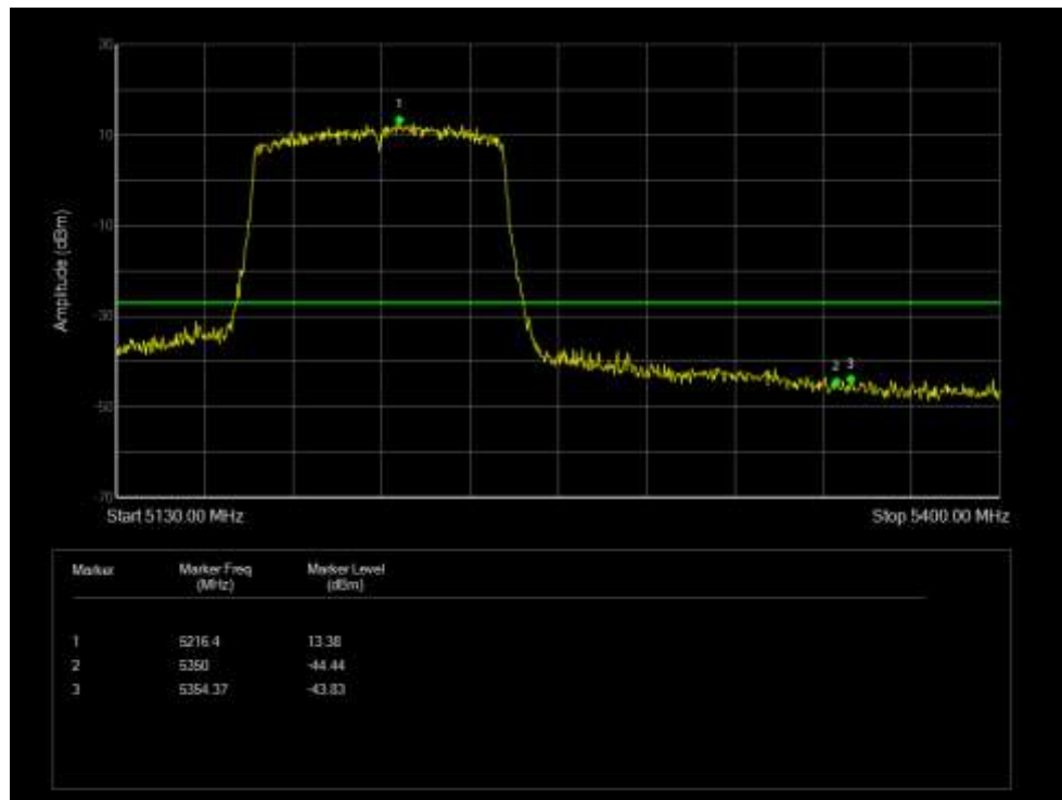
Band Edge NVNT 802.11ac80 5210MHz Low Ant 7
