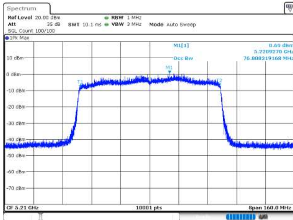
-26 dB BW NVNT 802.11ax80 5210MHz Ant 5
