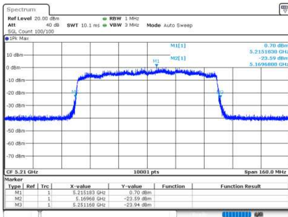
-26 dB BW NVNT 802.11ax80 5210MHz Ant 6
