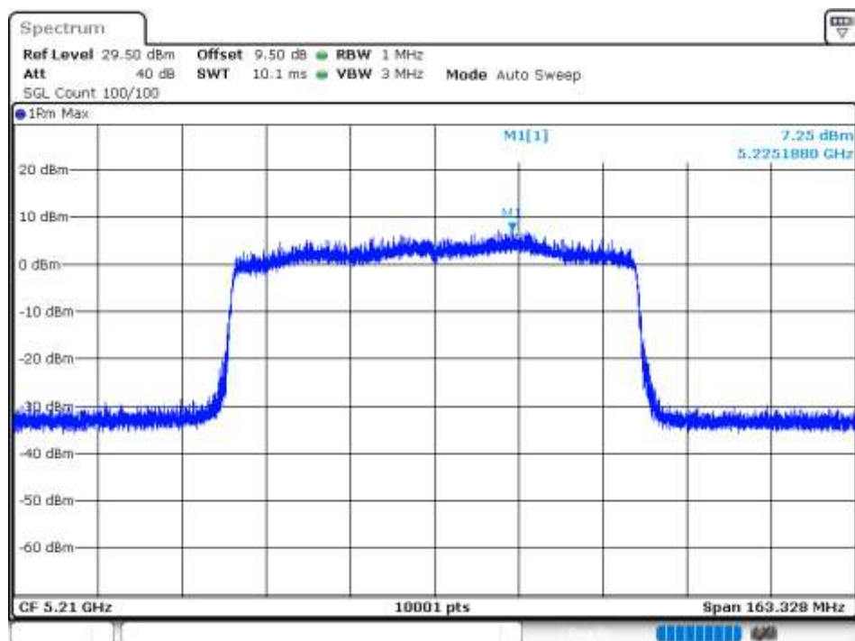
PSD NVNT 802.11ax80 5210MHz Ant 5
