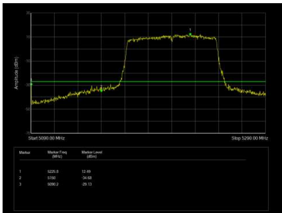
Band Edge NVNT 802.11ac80 5210MHz High Ant 5
