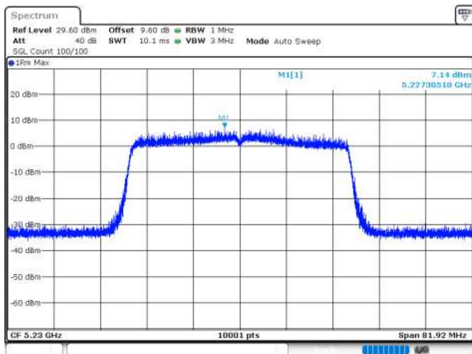
PSD NVNT 802.11ax40 5230MHz Ant 5
