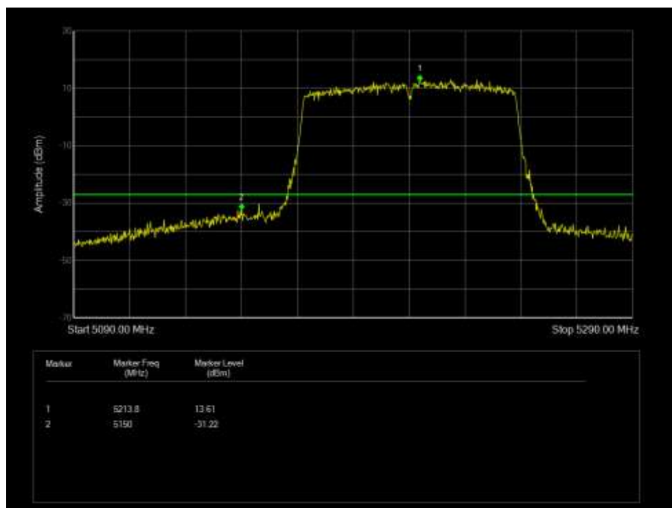
Band Edge NVNT 802.11ax20 5180MHz Low Ant 4
