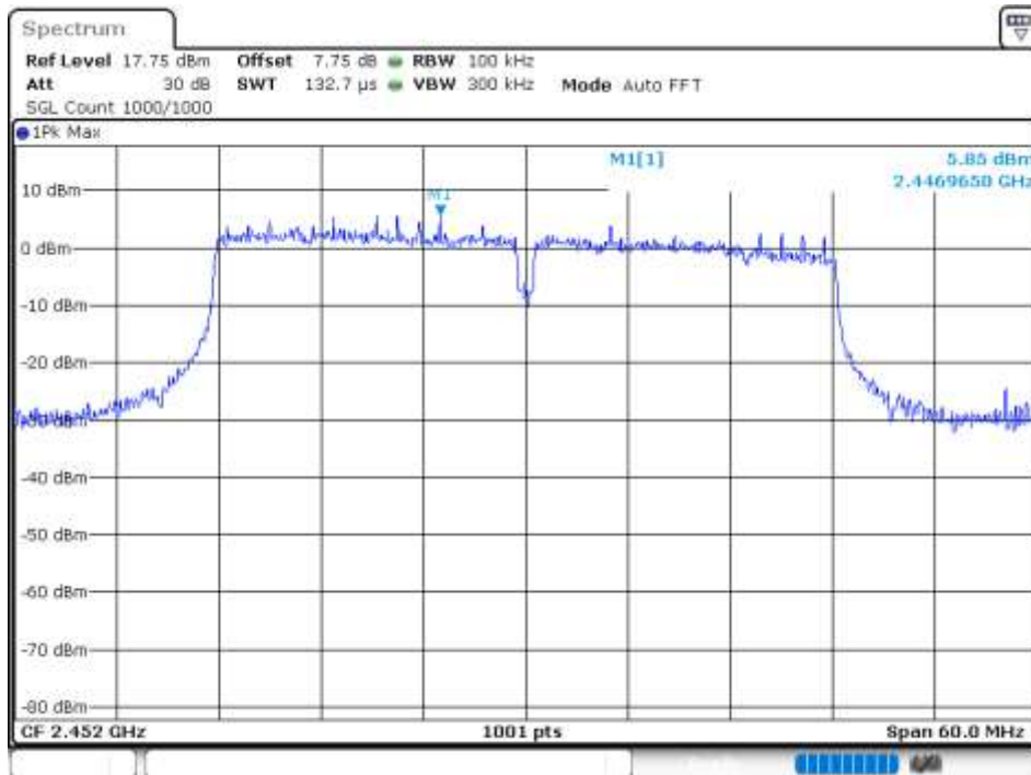
Band Edge NVNT 802.11n(HT40) 2452MHz Ant 0 Ref
