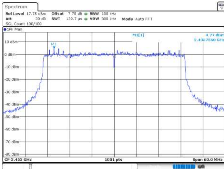
Band Edge NVNT 802.11ax40 2452MHz Ant 2 Ref
