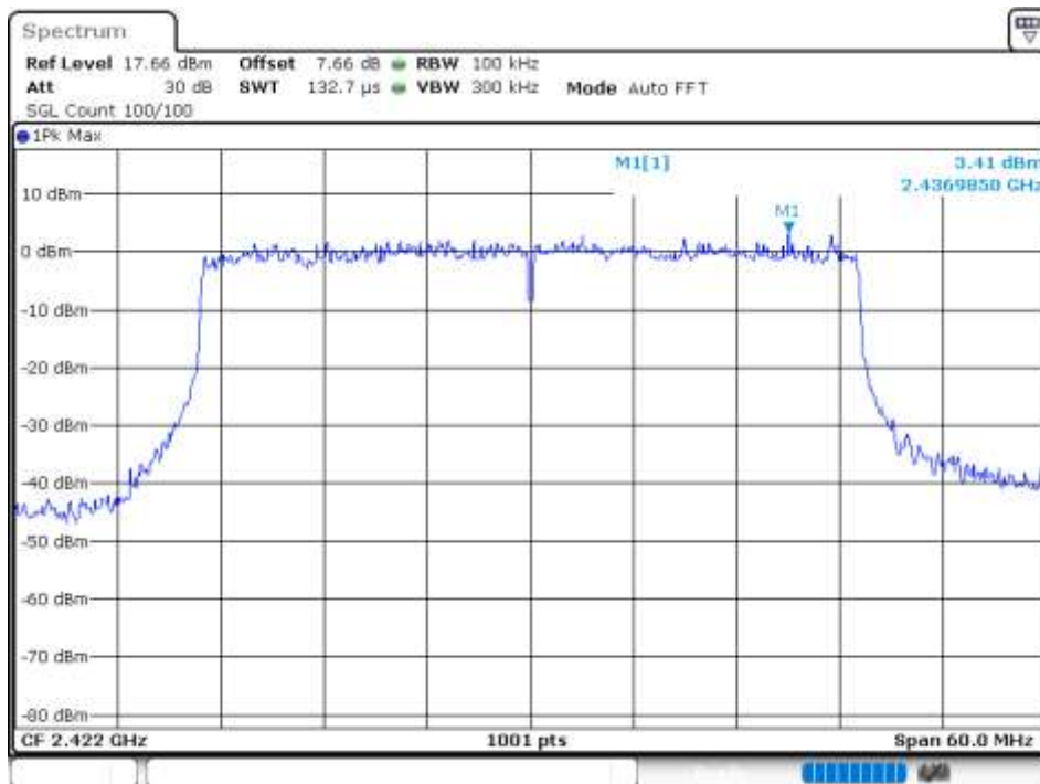
Band Edge NVNT 802.11ax40 2422MHz Ant 2 Ref
