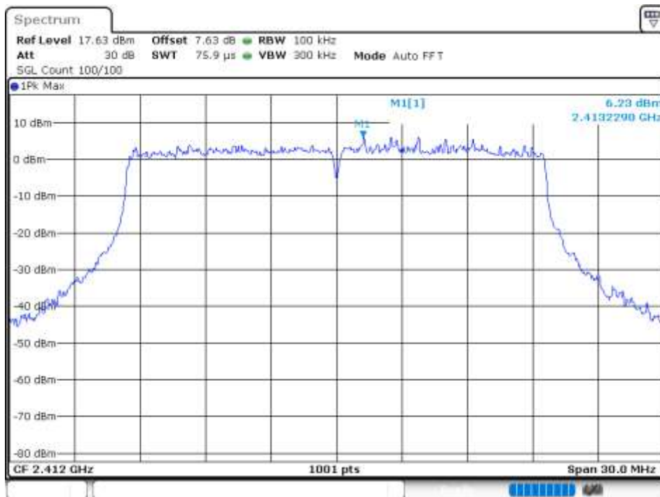
Band Edge NVNT 802.11ax20 2412MHz Ant 3 Ref
