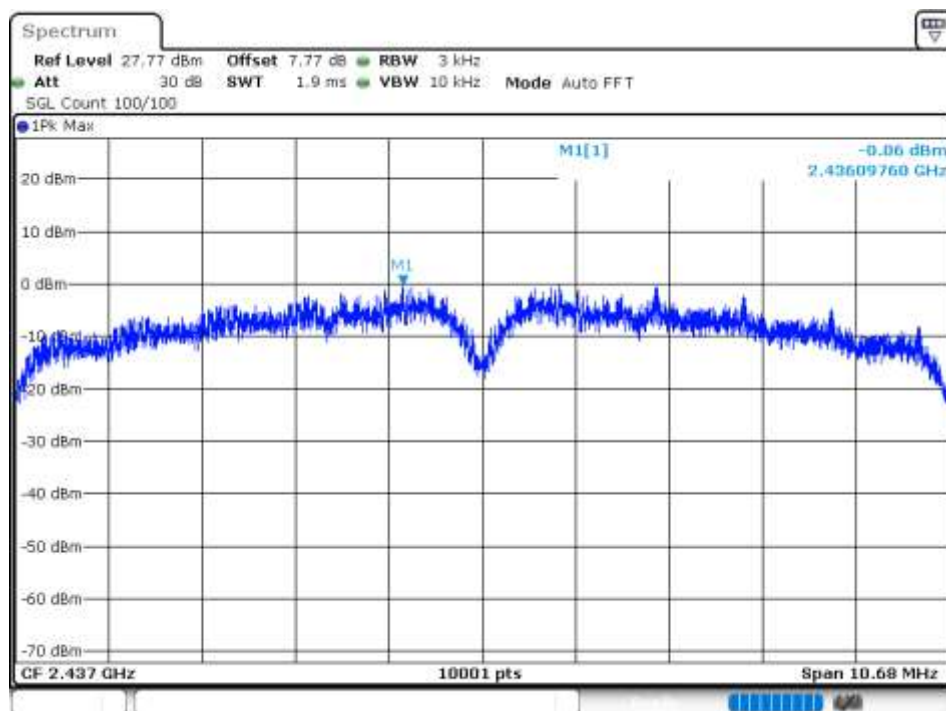
PSD NVNT 802.11b 2437MHz Ant 3
