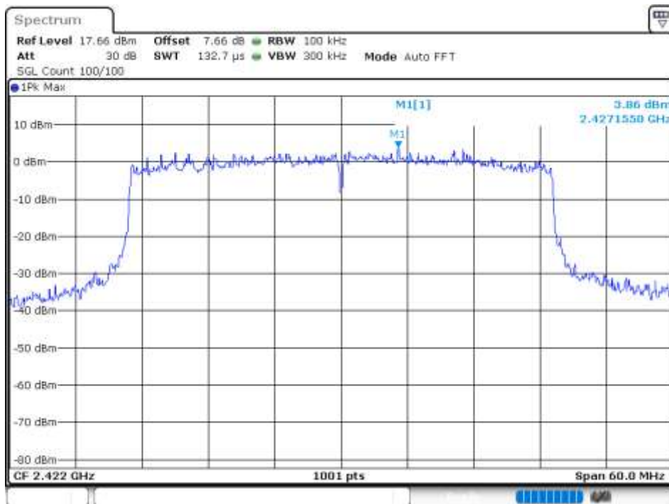
Band Edge NVNT 802.11ax40 2422MHz Ant 1 Ref
