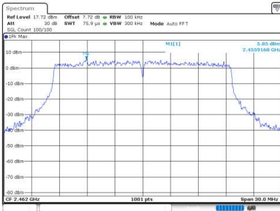
Band Edge NVNT 802.11ax20 2462MHz Ant 3 Ref
