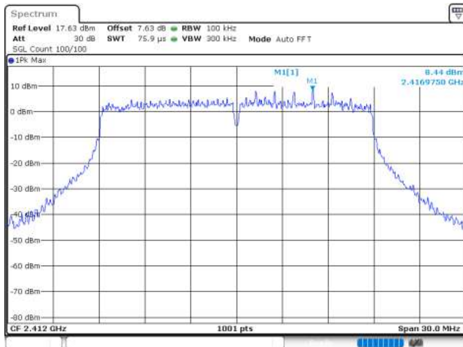
Band Edge NVNT 802.11n(HT20) 2412MHz Ant 3 Ref
