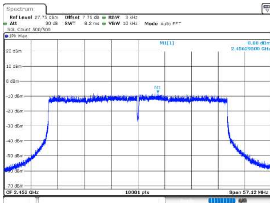
PSD NVNT 802.11ax40 2452MHz Ant 2
