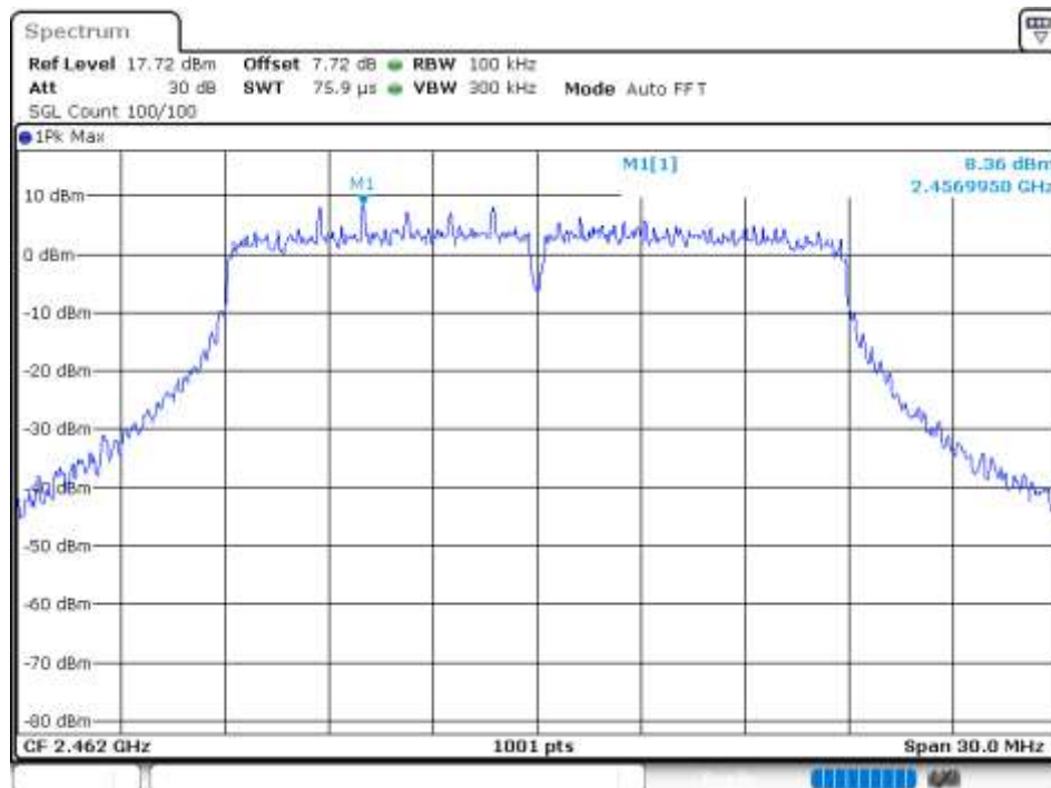
Band Edge NVNT 802.11n(HT20) 2462MHz Ant 3 Ref
