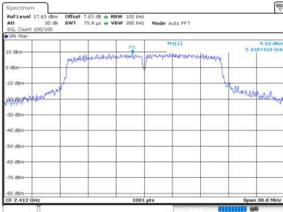
Band Edge NVNT 802.11g 2412MHz Ant 0 Ref
