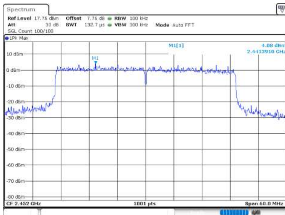
Band Edge NVNT 802.11ax40 2452MHz Ant 1 Ref
