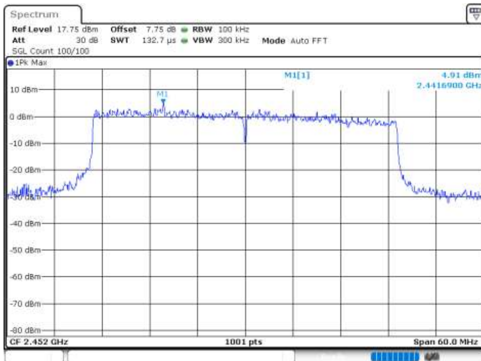
Band Edge NVNT 802.11ax40 2452MHz Ant 0 Ref
