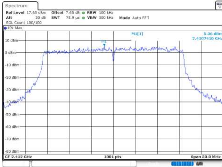
Band Edge NVNT 802.11ax20 2412MHz Ant 0 Ref
