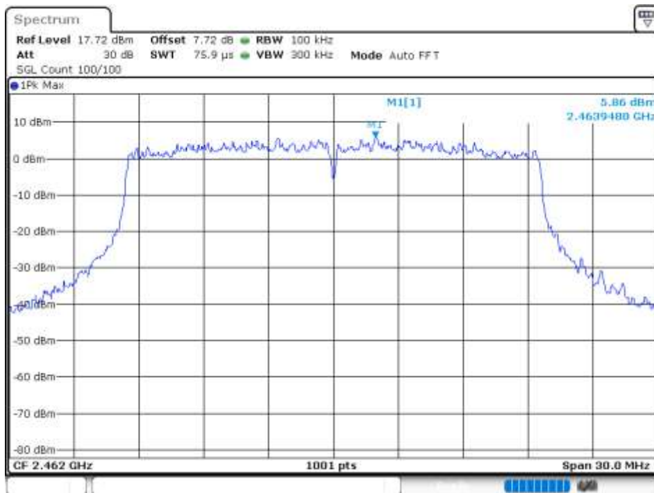
Band Edge NVNT 802.11ax20 2462MHz Ant 2 Ref
