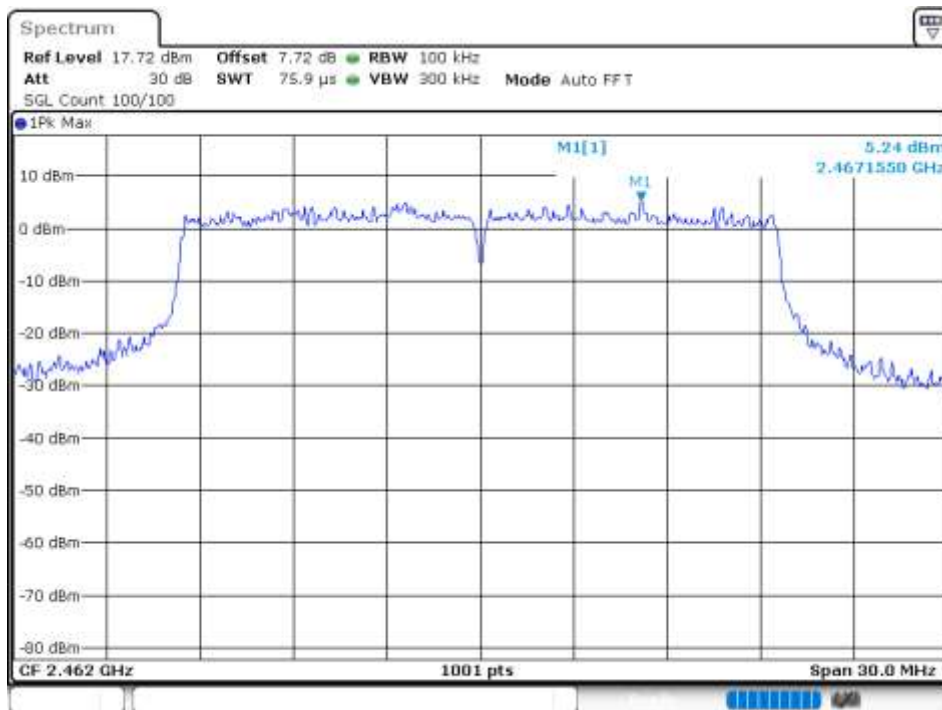
Band Edge NVNT 802.11ax20 2462MHz Ant 1 Ref
