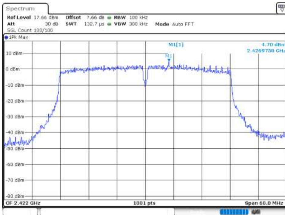
Band Edge NVNT 802.11n(HT40) 2422MHz Ant 0 Ref
