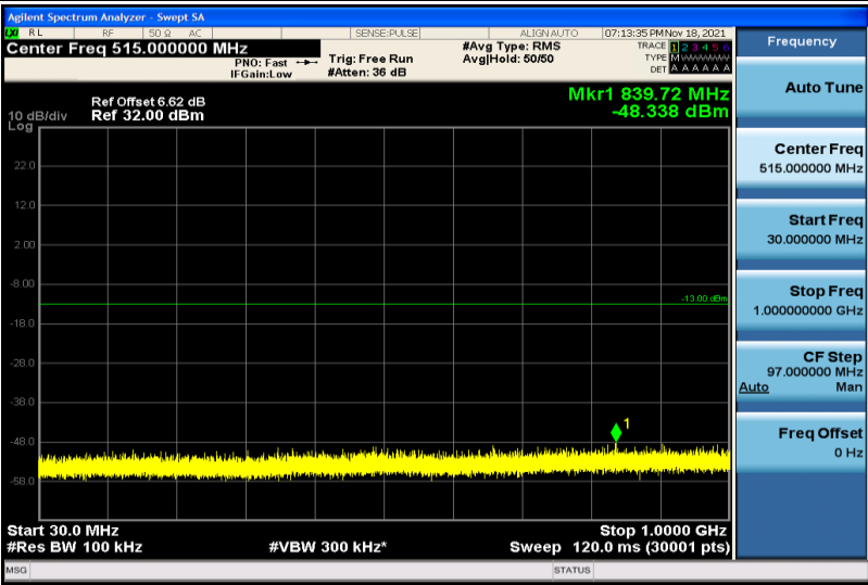
Band4-3MHz-QPSK-20385-1RB#0-30~1000MHz
