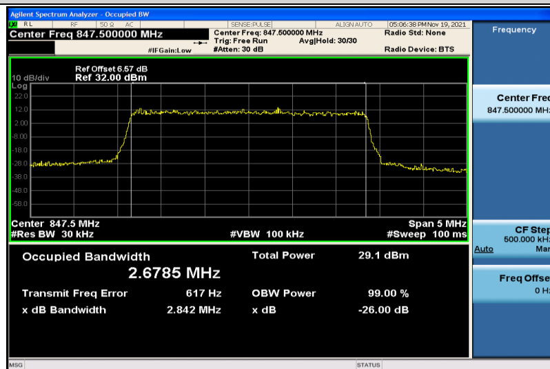
Band5-3MHz-QPSK-20635-15RB#0-2.6785
