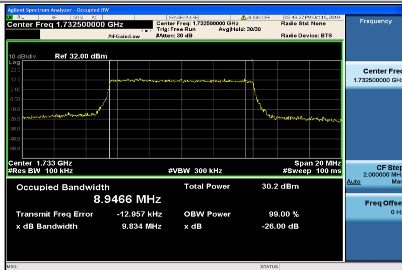
Band4-10MHz-QPSK-20175-50RB#0-8.9466
