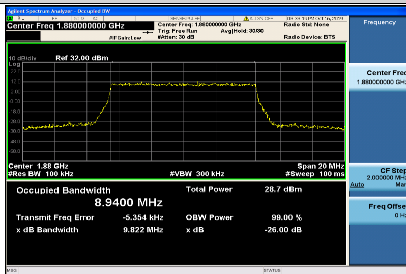
Band2-10MHz-QPSK-18900-50RB#0-8.9400
