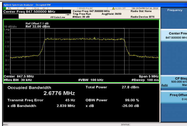
Band5-3MHz-QPSK-20635-15RB#0-2.6776
