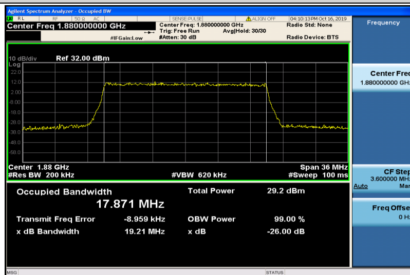
Band2-20MHz-QPSK-18900-100RB#0-17.871
