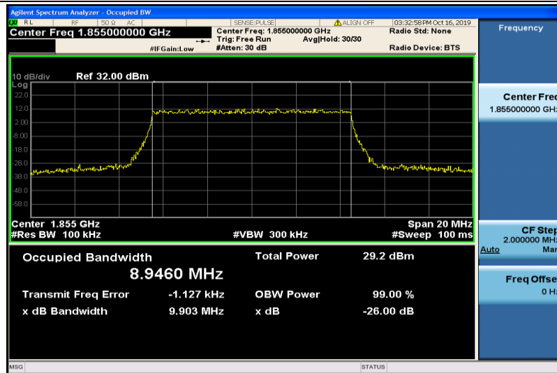
Band2-10MHz-QPSK-18650-50RB#0-8.9460
