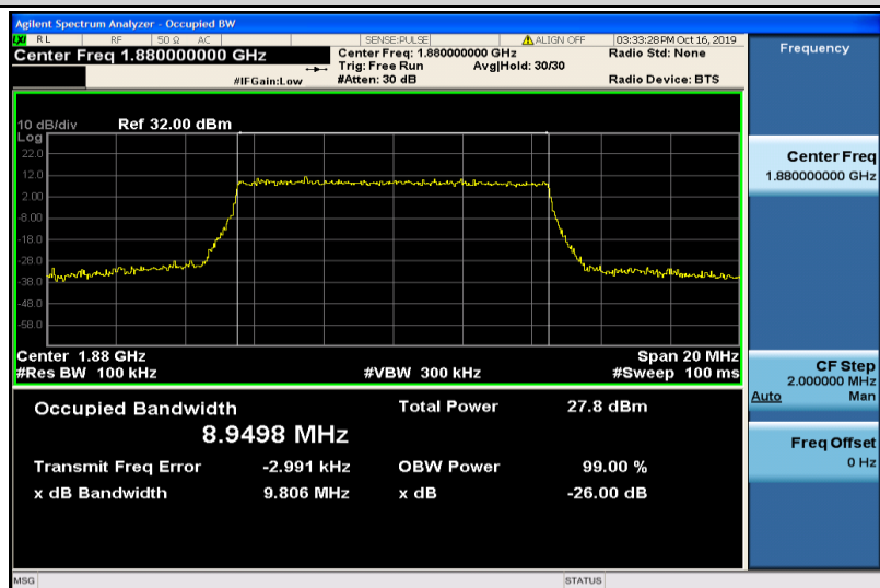
Band2-10MHz-16QAM-18900-50RB#0-8.9498
