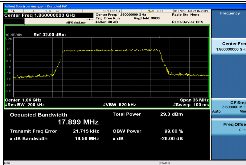
Band2-20MHz-QPSK-18700-100RB#0-17.899
