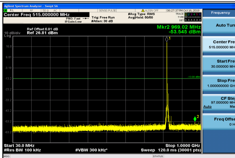
Band5-5MHz-QPSK-20425-1RB#0-30~1000MHz
