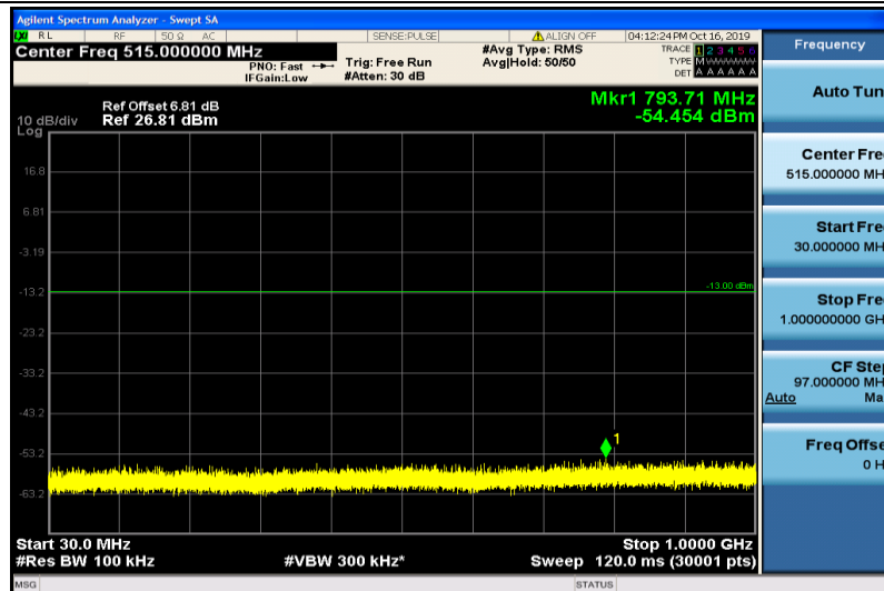
Band2-20MHz-QPSK-18700-1RB#0-30~1000MHz
