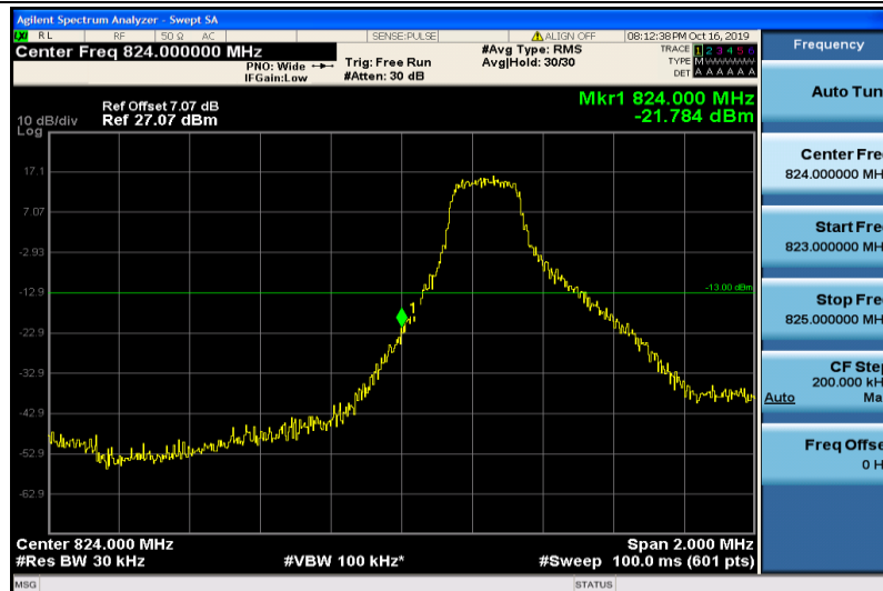
Band5-3MHz-QPSK-20415-1RB#0
