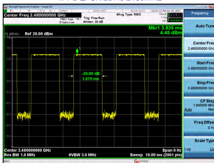
\pi/4 -DQPSK 2DH3 2480MHZ
