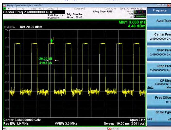
\pi/4 -DQPSK 2DH1 2480MHZ
