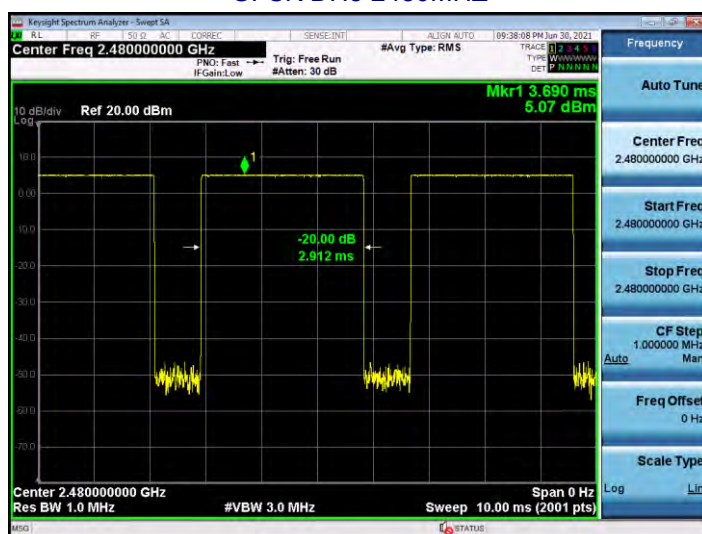
GFSK DH5 2480MHZ
