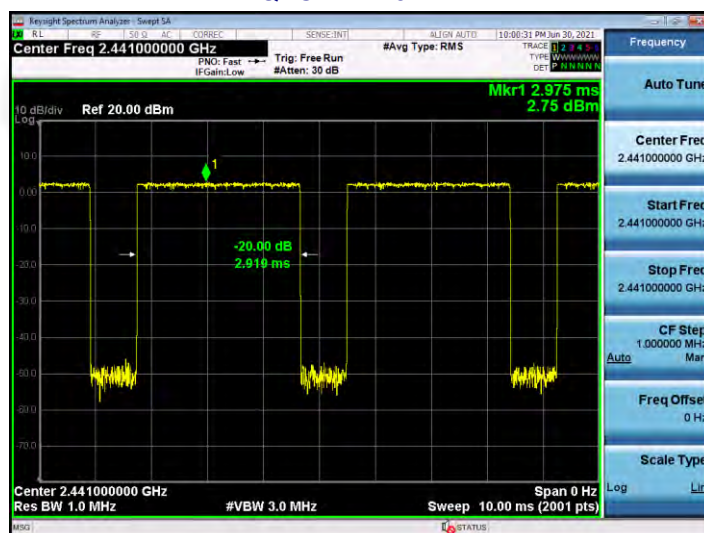
\pi/4 -DQPSK 2DH5 2441MHZ
