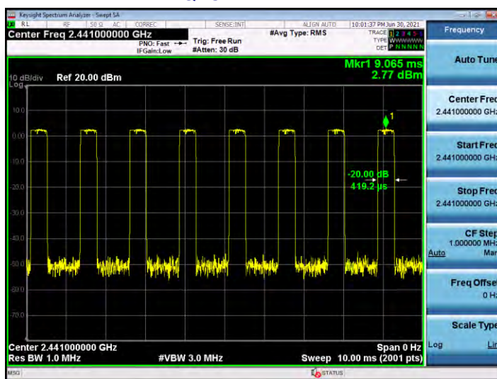
\pi/4 -DQPSK 2DH1 2441MHZ
