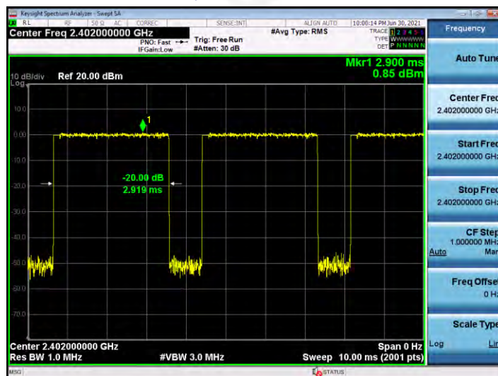
\pi/4 -DQPSK 2DH5 2402MHZ
