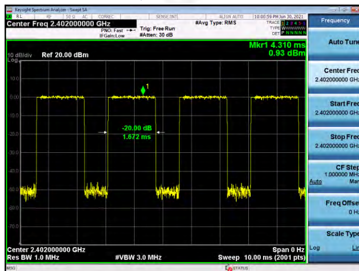
\pi/4 -DQPSK 2DH3 2402MHZ
