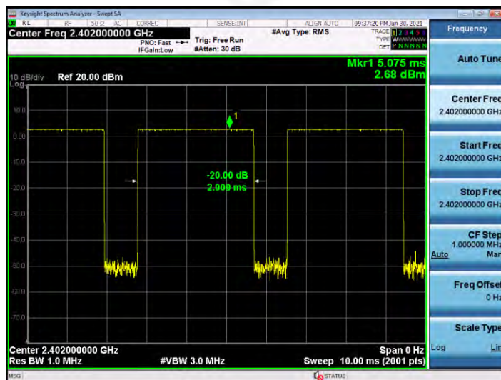
GFSK DH5 2402MHZ
