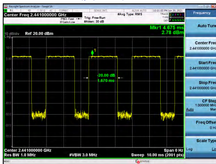
\pi/4 -DQPSK 2DH3 2441MHZ
