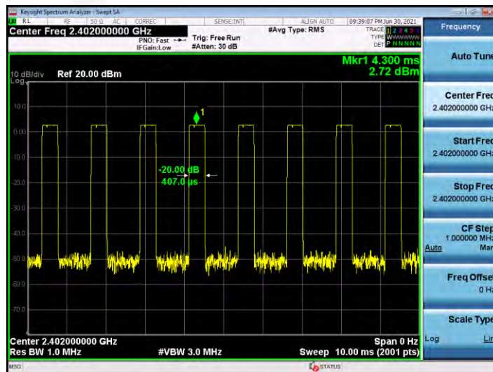
GFSK DH1 2402MHZ
