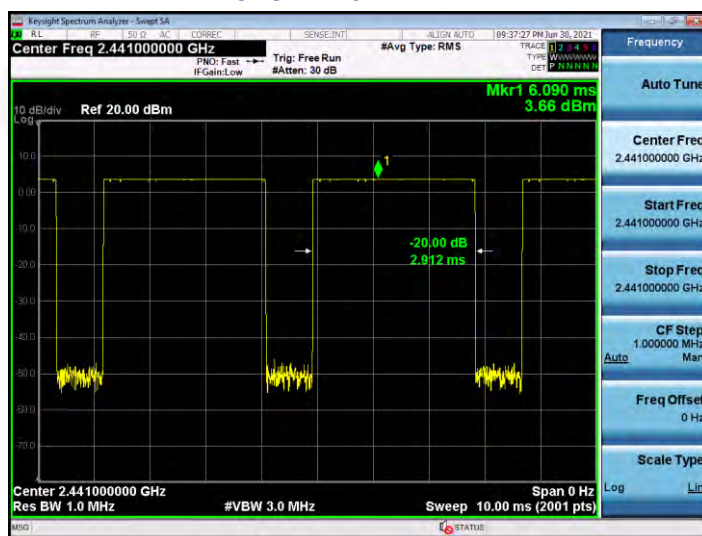
GFSK DH5 2441MHZ
