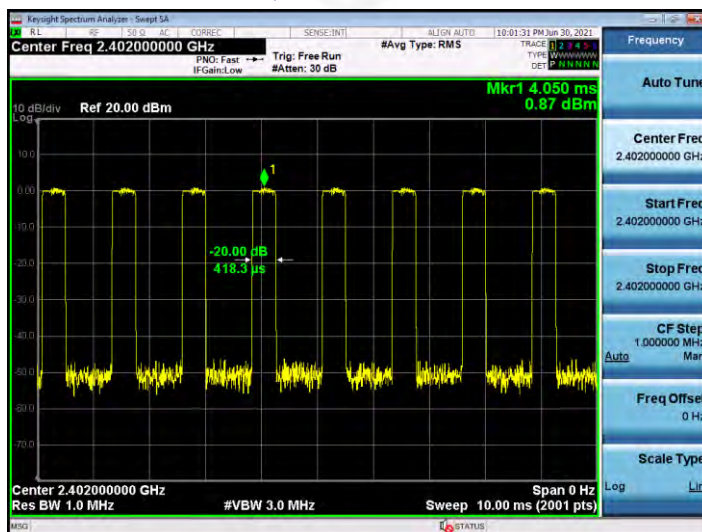
\pi/4 -DQPSK 2DH1 2402MHZ
