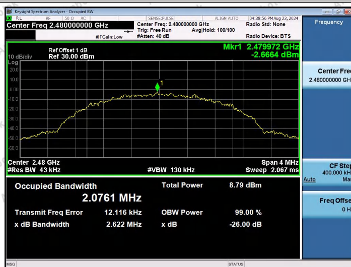
BLE_2M-Ant1-2480
