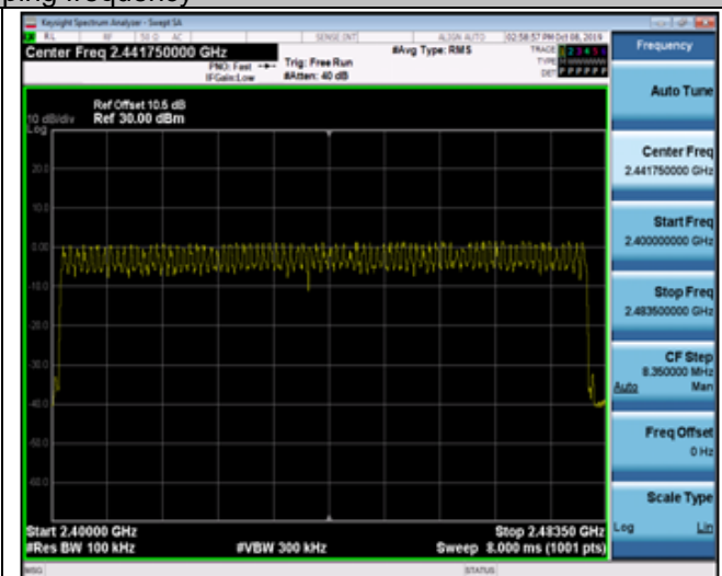
\pi/4 -DQPSK
