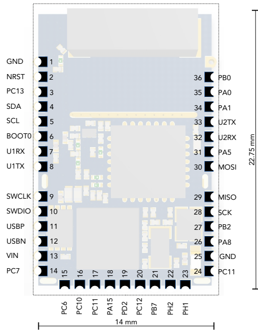
FMLR-72-C-STL0Z-(4M)
